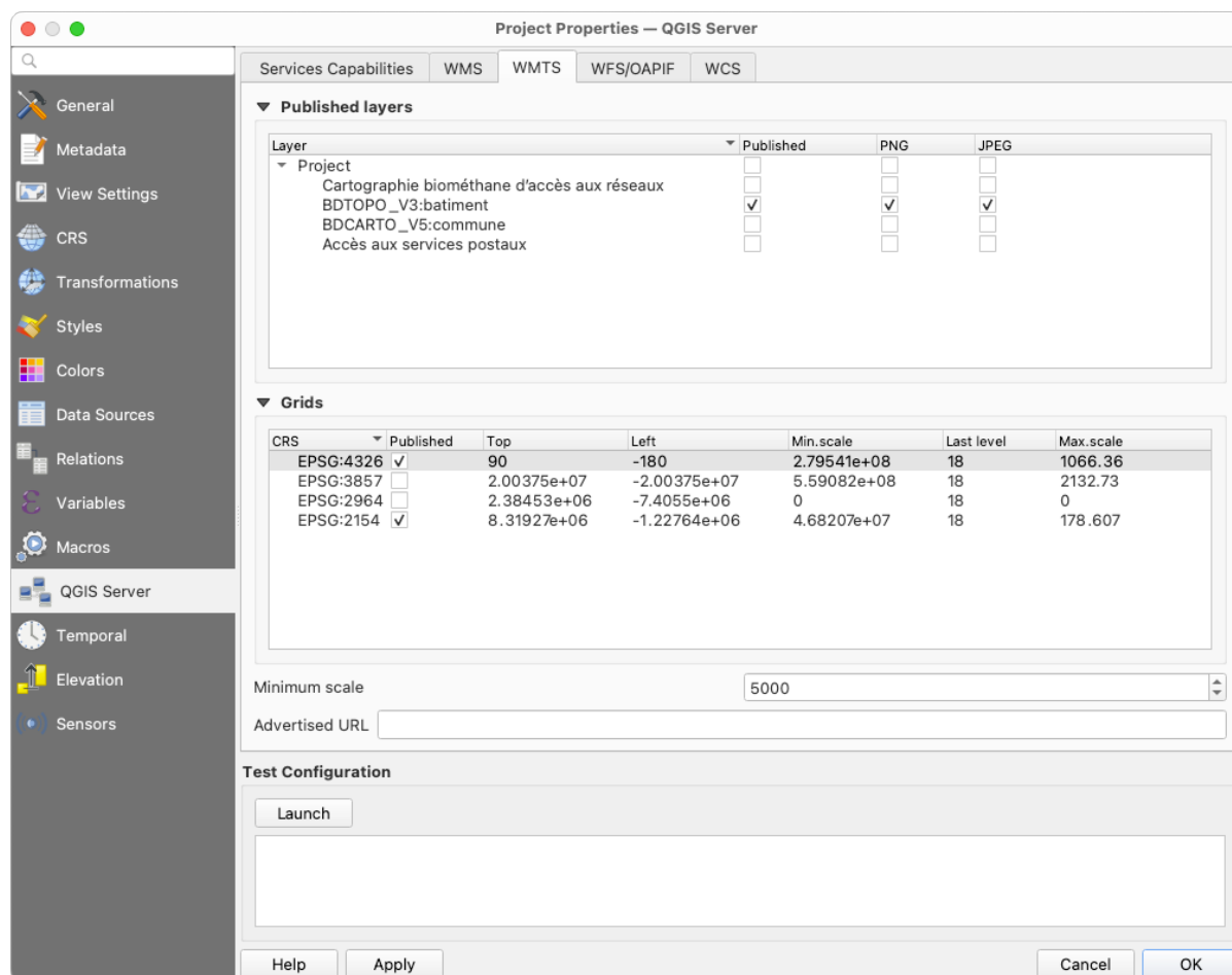
Fig. 2.4: Definities op de tab WMTS
