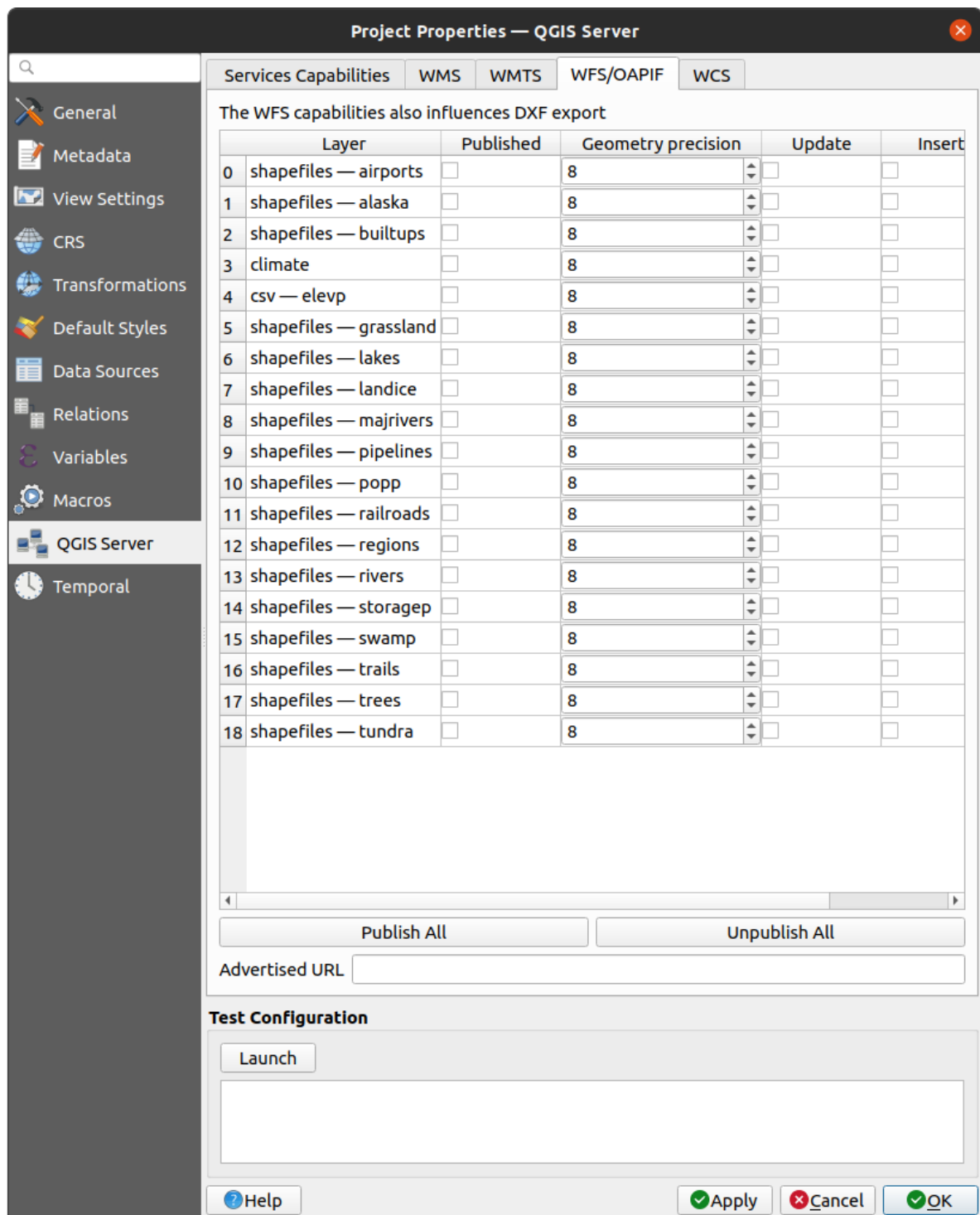
Fig. 2.5: Definities op de tab WFS/OAPIF
