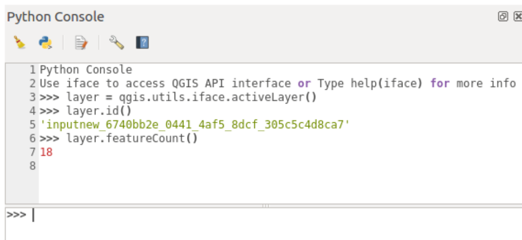
1.1 Fig. : QGIS Python konsolè
