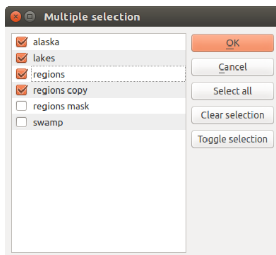
Fig. 27.14: Selecție Multiplă
