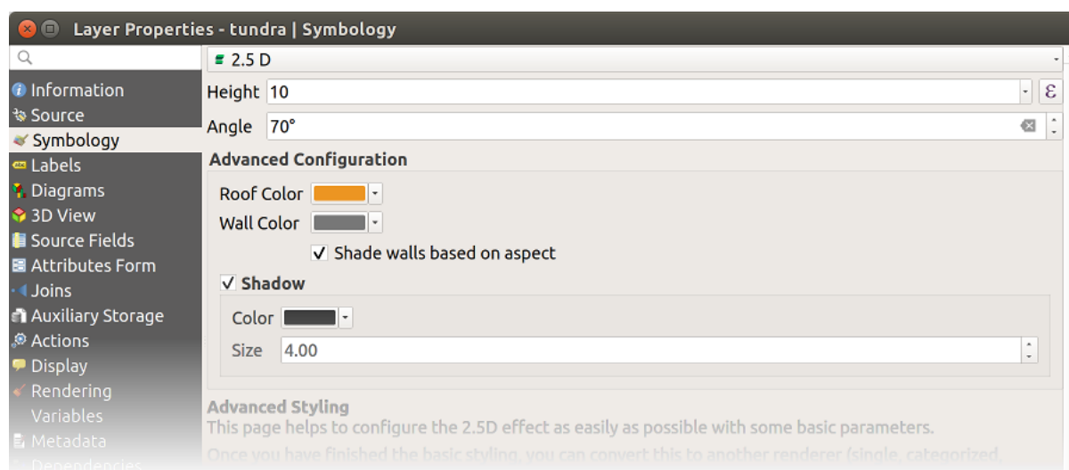
Fig. 16.12: 2.5D dialog
