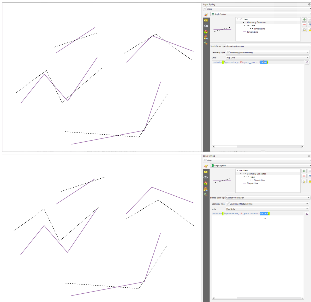
Fig. 13.7: Objecten roteren
