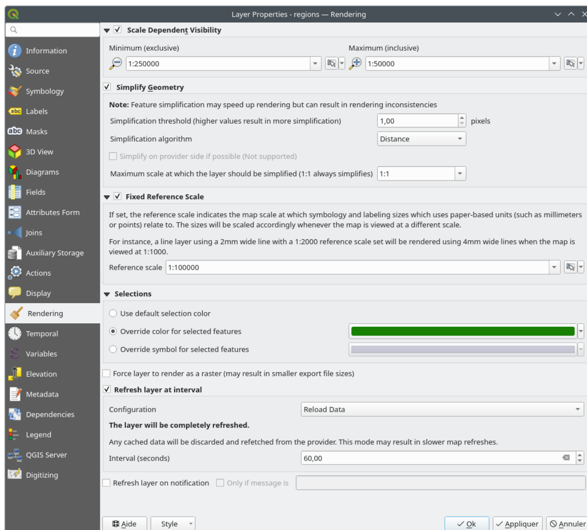
Fig. 16.60: Dialoogvenster Laageigenschappen
