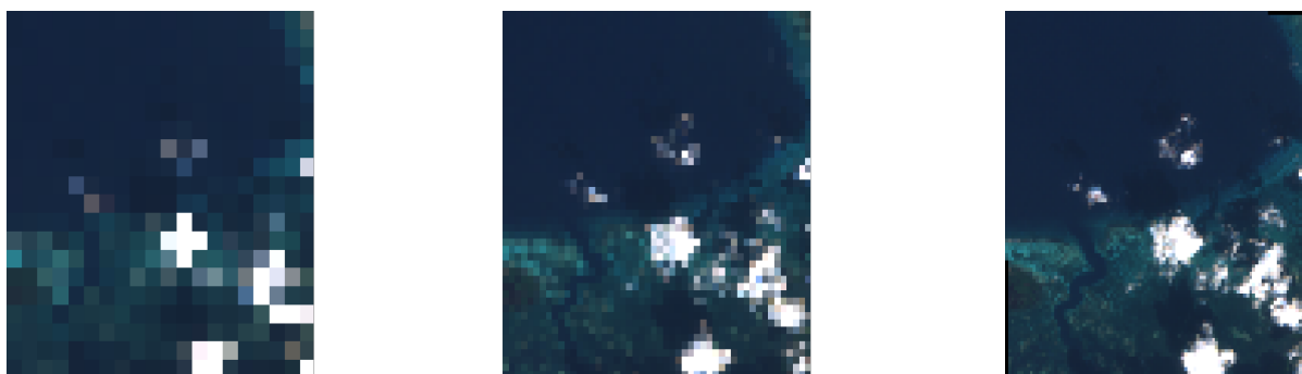
図 3.23: 左から、WIDTH=20&HEIGHT=20、WIDTH=50&HEIGHT=50、WIDTH=100&HEIGHT=100
