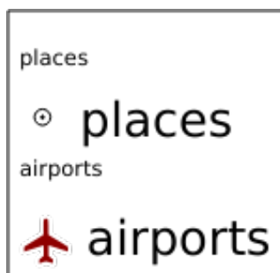
図 3.18: ITEMFONTSIZE=30 の凡例
