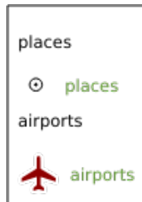
図 3.20: ITEMFONTCOLOR=0x5f9930 の凡例
