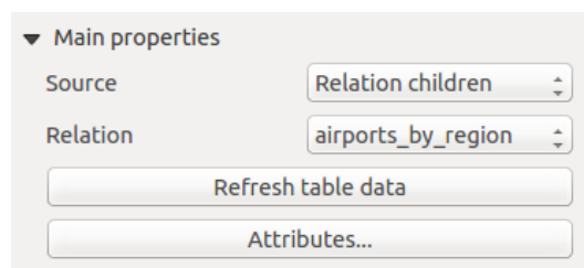
Figure22.41: Propriétés principales d'une Table d'attributs pour les "Enfants d'une Relation"
