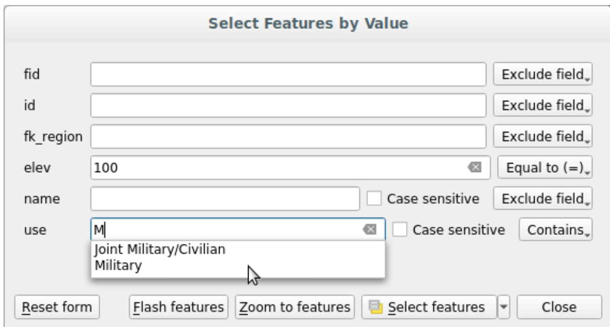
Figure12.10: Filtrer / sélectionner des entités à l’aide de la boîte de dialogue du formulaire
