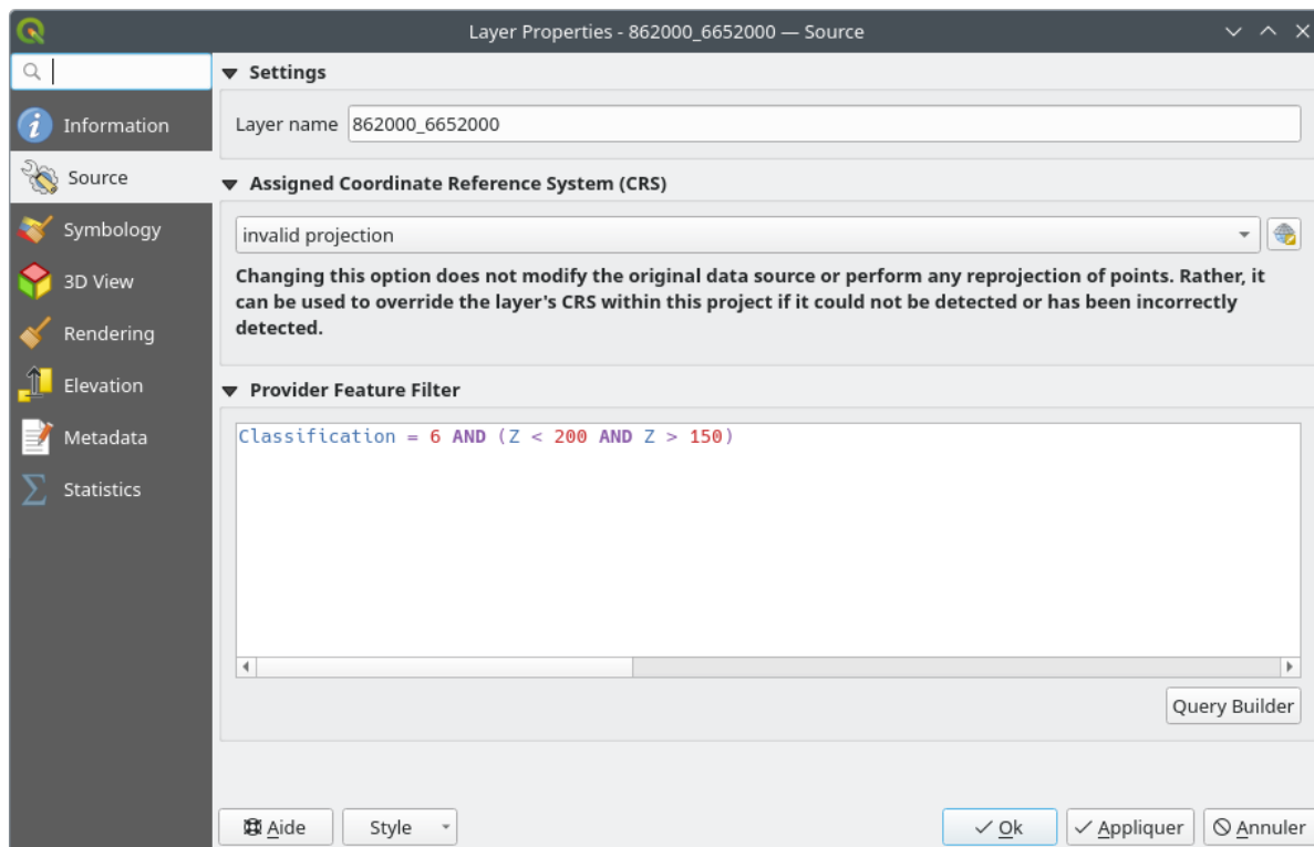
Figure20.2: Onglet source de nuage de points
