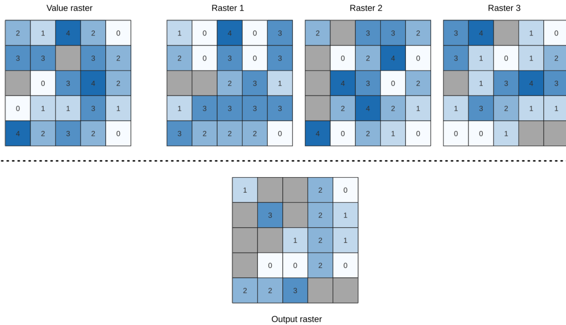
Figura 28.25: Para cada celda del ráster de salida, el valor representa la cantidad de veces que las celdas correspondientes en la lista de rásteres son menores que el ráster de valor. Se tienen en cuenta las celdas NoData (grises).
