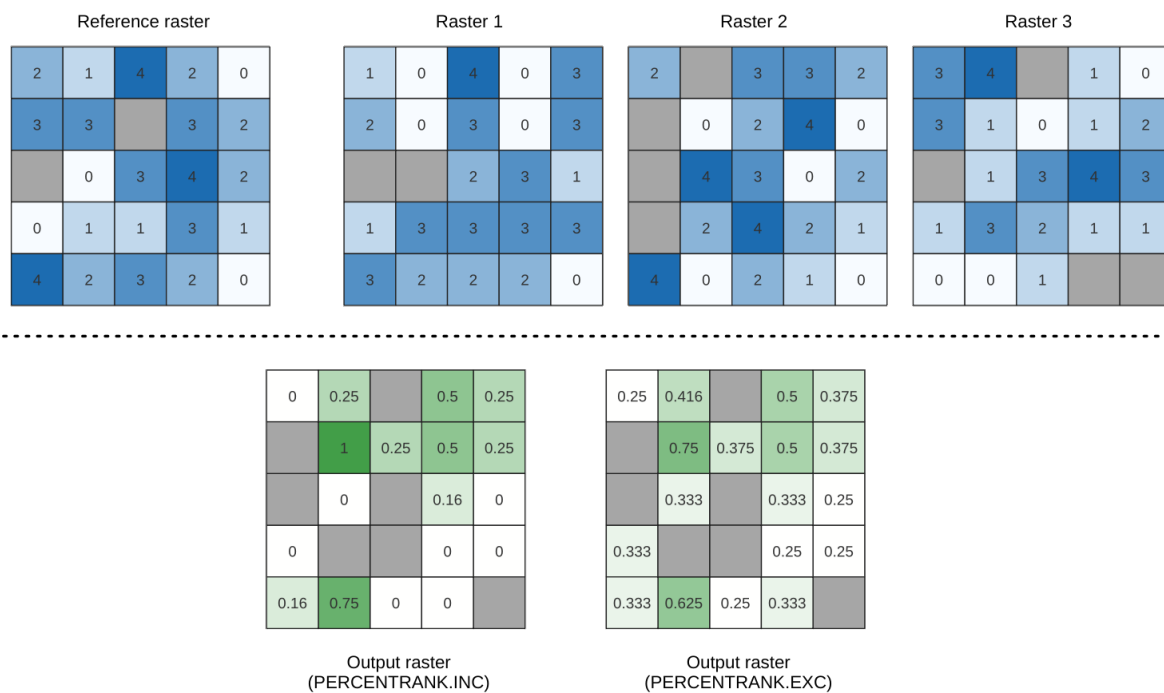
Figura 28.18: Clasificación porcentual Valor = 1. Las celdas NoData (grises) se ignoran.
