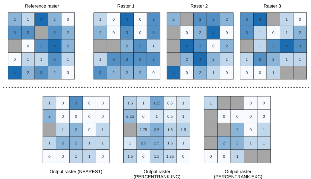
Figura 28.19: Percentil = 0,25. Las celdas NoData (grises) se ignoran.
