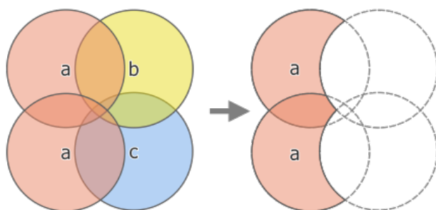
Figura 28.120: Operación de diferencia entre una capa de entrada de dos características “a” y capas superpuestas de una sola característica “b” y “c” (izquierda), lo que da como resultado una nueva capa con las características “a” modificadas (derecha)
