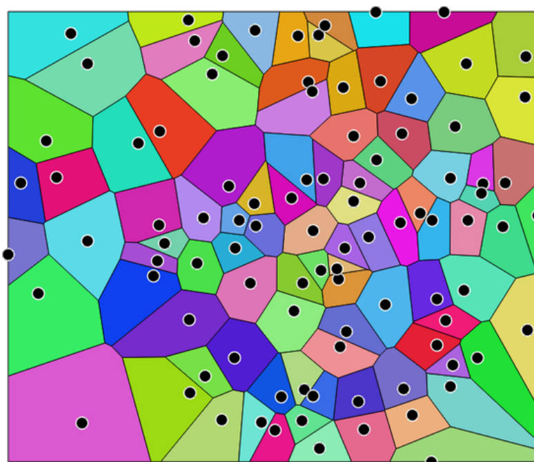
Figura 28.117: Polígonos Voronoi
