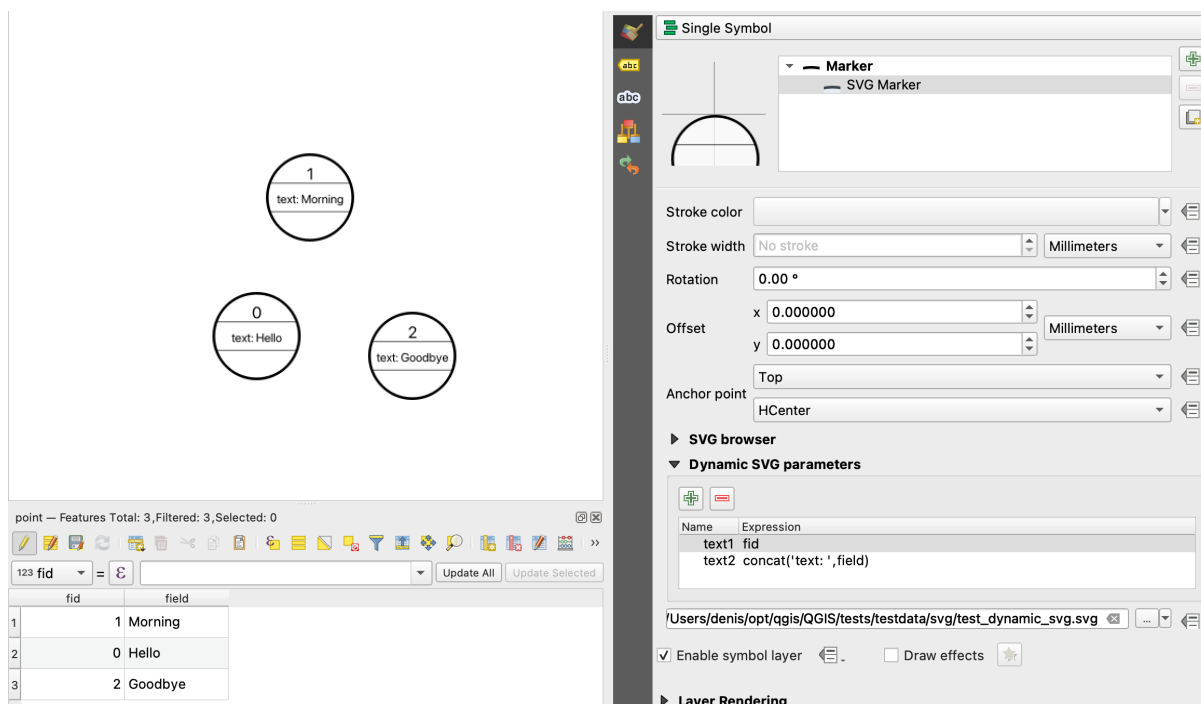
Obr. 14.20: Dynamic SVG parameters table
