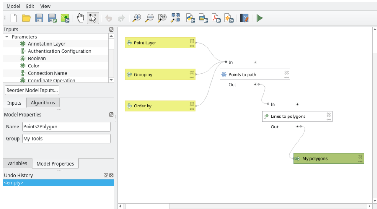
Obr. 27.2: Modelář zpracování
