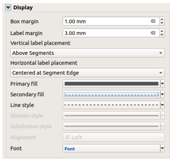
Рис. 21.37: Scale Bar Display group
