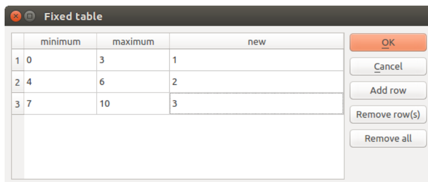
Рис. 26.14: Fixed Table
