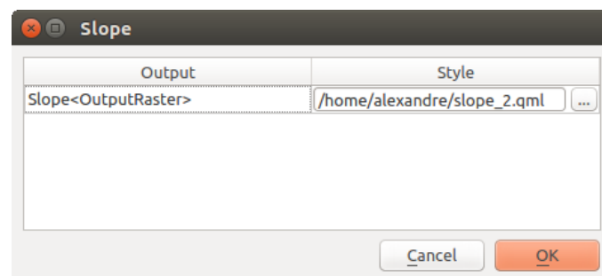
Рис. 26.5: Rendering Styles
