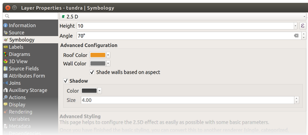
Рис. 16.12: 2.5D dialog
