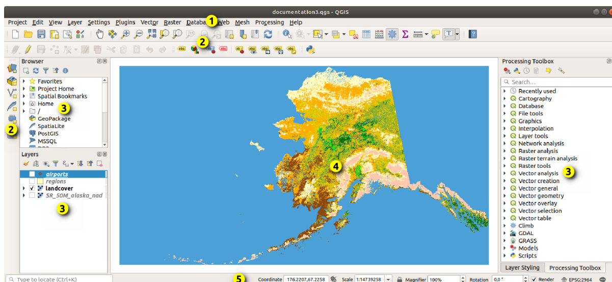
Рис. 11.1: QGIS GUI
