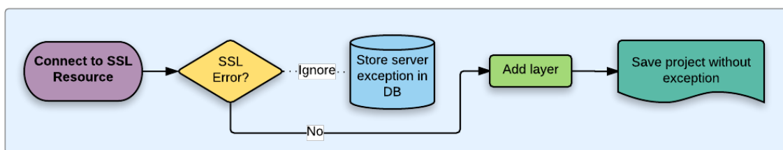
Рис. 24.35: SSL server exception
