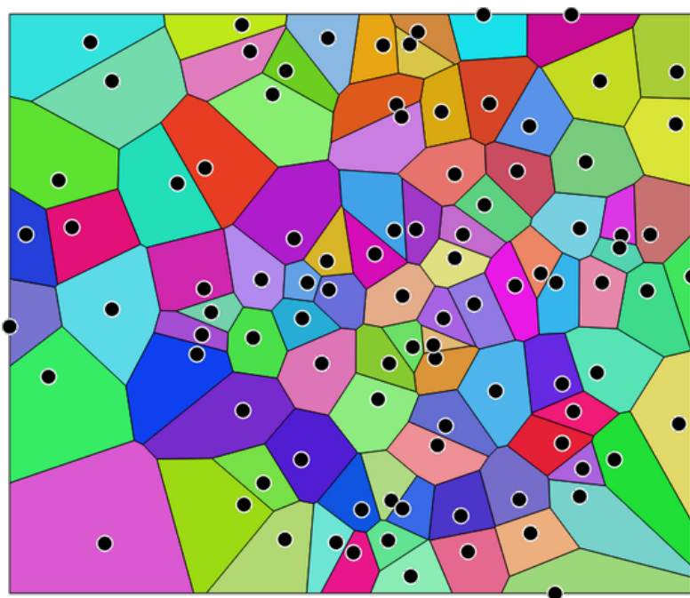
Рис. 27.108: Voronoi polygons
