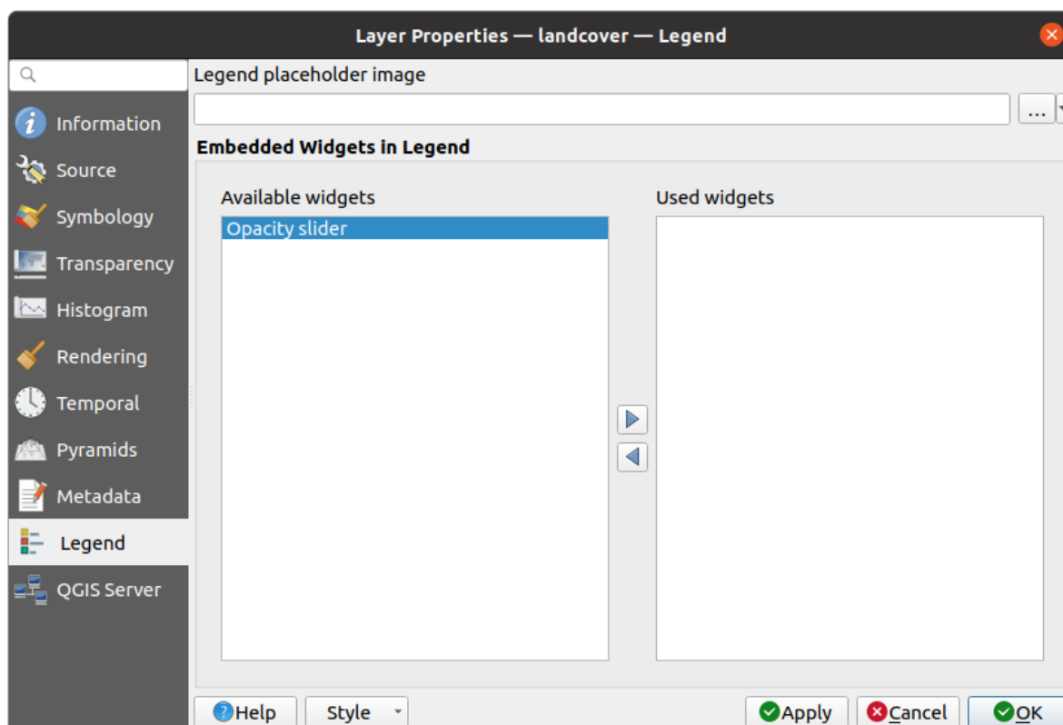
Рис. 17.19: Raster Legend
