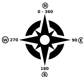
Рис. 27.21: Aspect values
