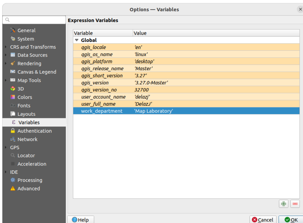
Рис. 9.20: Variables settings
