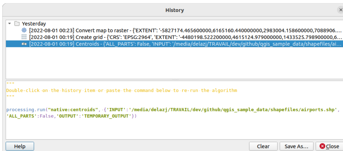
Рис. 26.16: History
