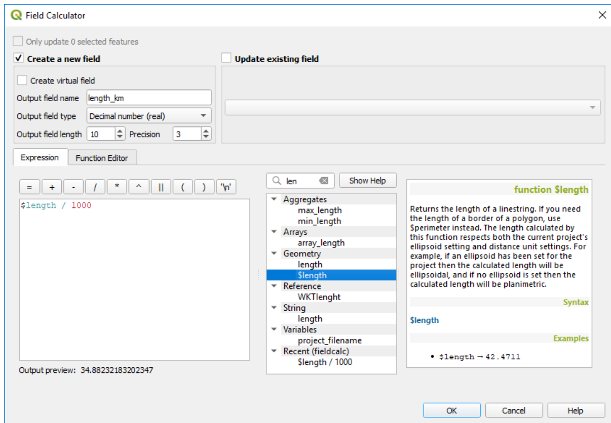
Fig. 16.72: Calculatorul de Câmpuri
