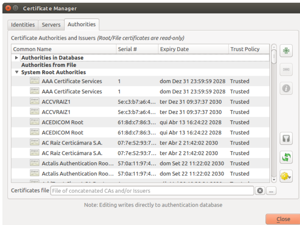
Fig. 24.24: Editorul de autorități
