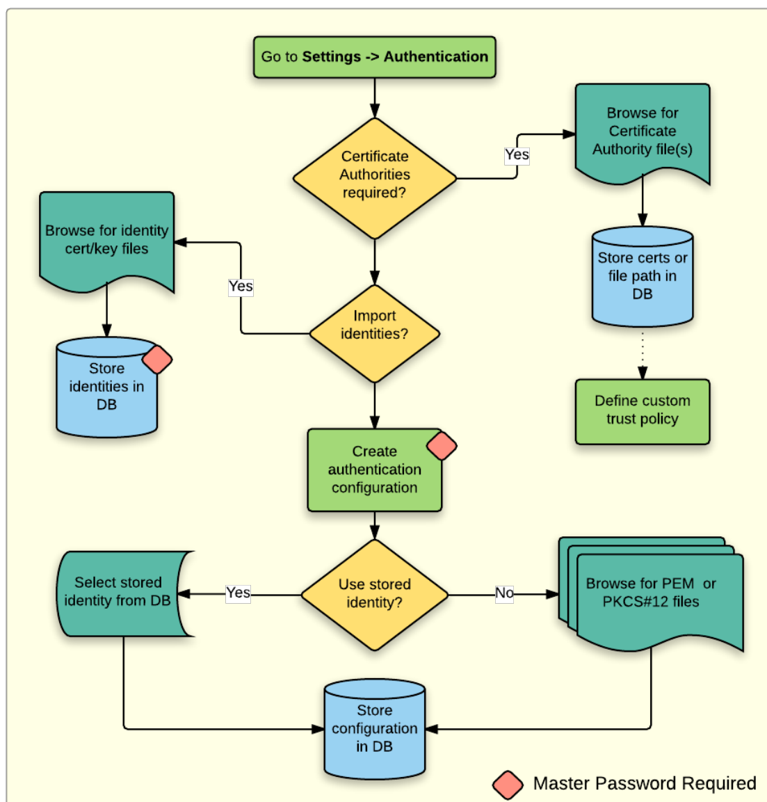
Fig. 24.22: Fluxul de lucru pentru configurarea PKI
