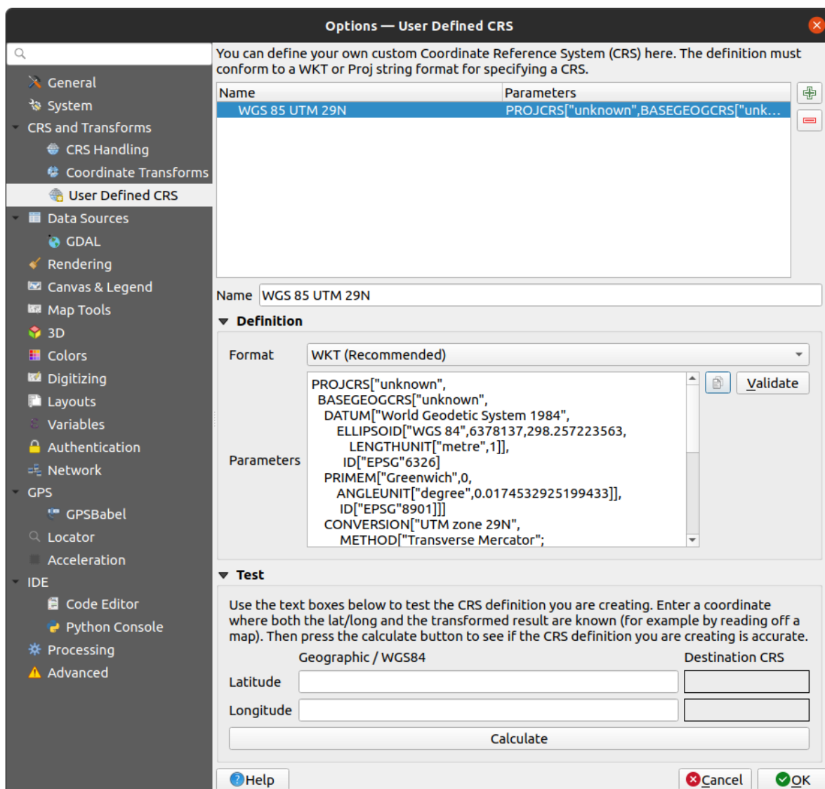
Fig. 10.3: Dialogul CRS-urilor Personalizate
