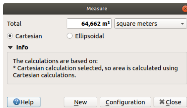
Fig. 11.16: Măsurarea Ariei
