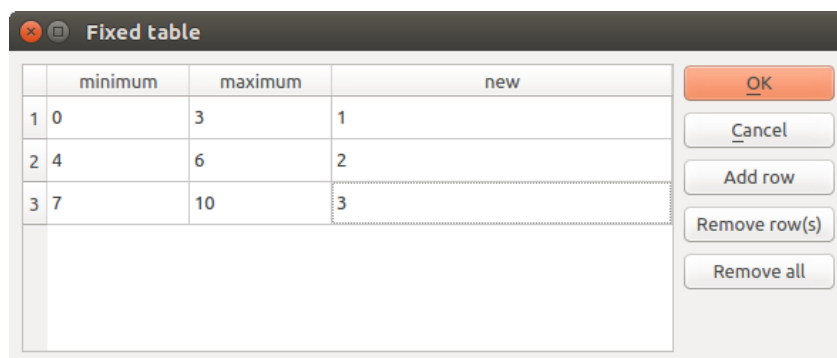
Fig. 26.14: Tabelă Reparată
