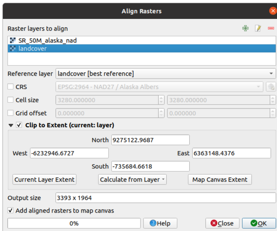
Fig. 17.23: Alinierea Rasterelor
