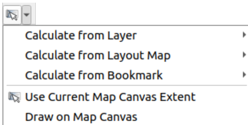
Fig. 26.12: Selectorul Extinderii
