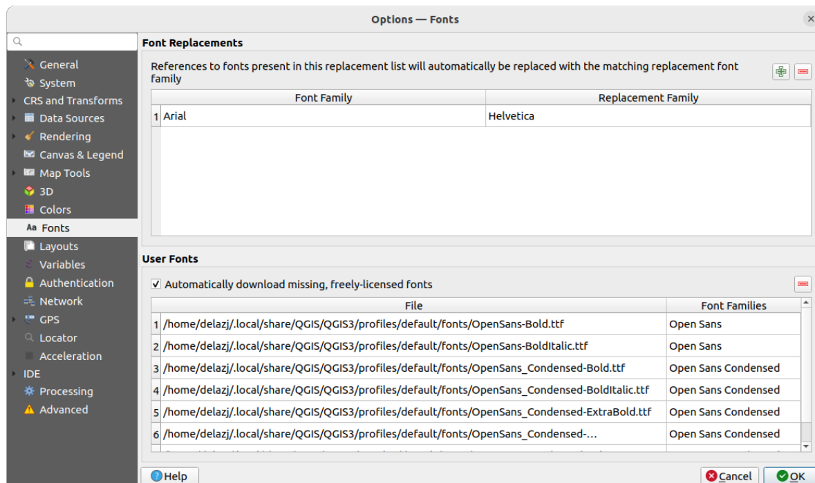
Fig. 9.18: Setările fonturilor
