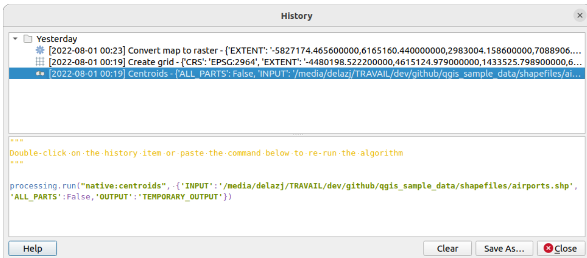
Fig. 26.3: Istoricul Processing
