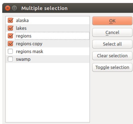
Fig. 26.13: Selecție Multiplă
