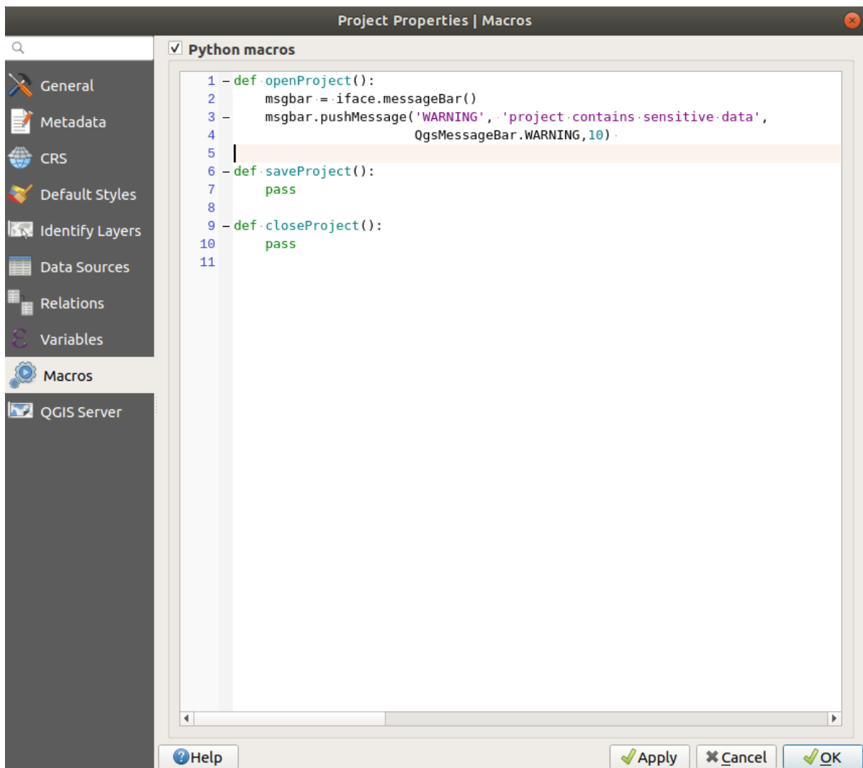
Fig. 9.36: Setări macro
