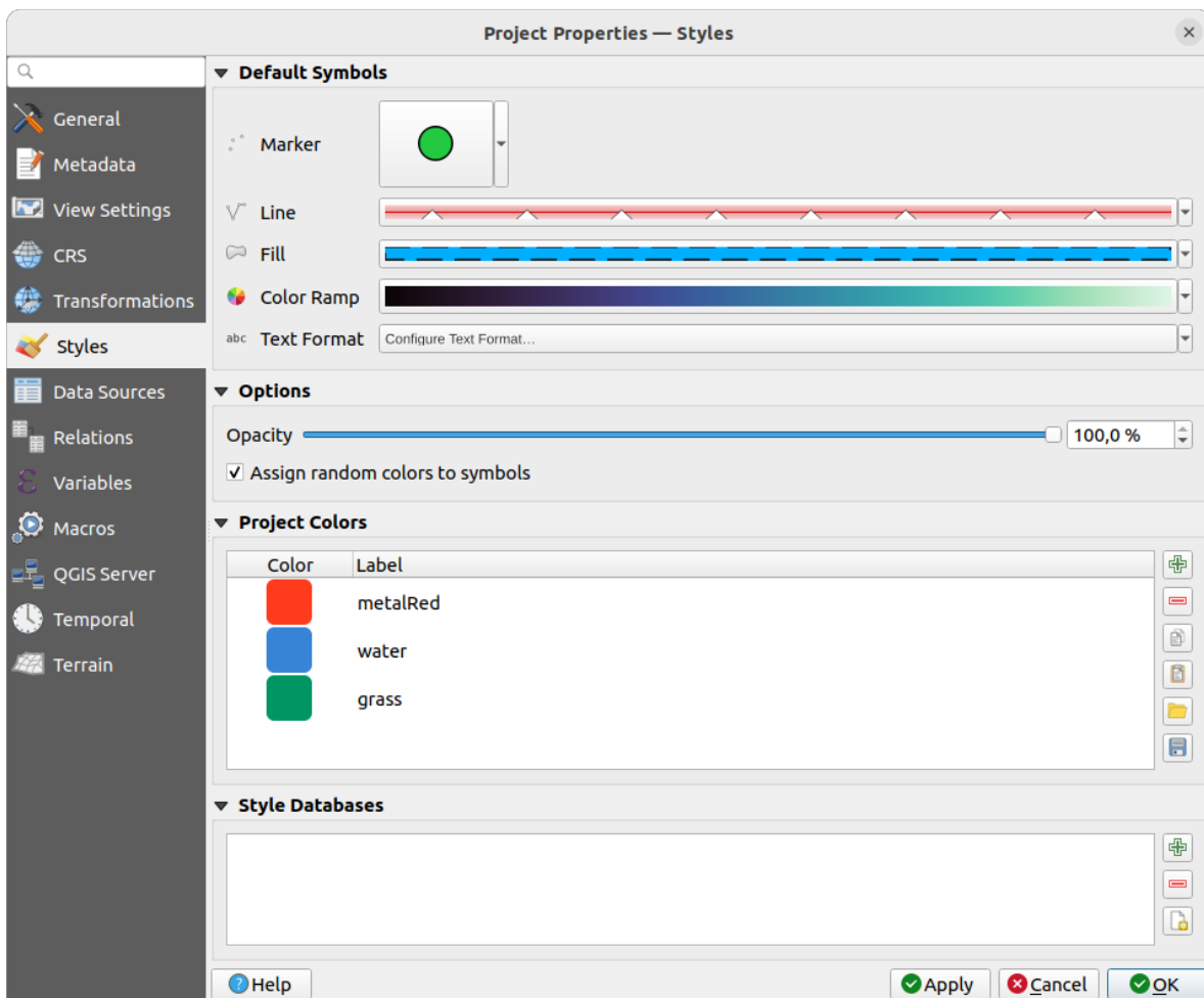
Fig. 9.33: Styles tab
