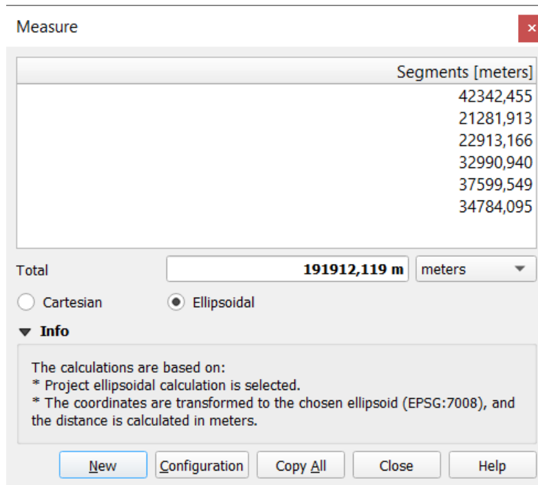
Fig. 11.15: Măsurarea Distanței
