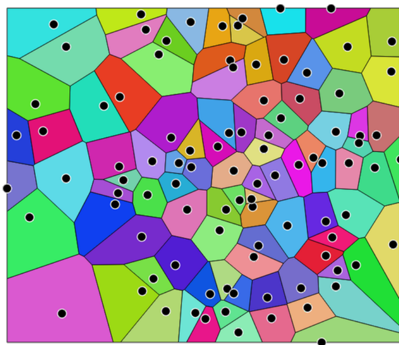
Fig. 27.108: Voronoi polygons
