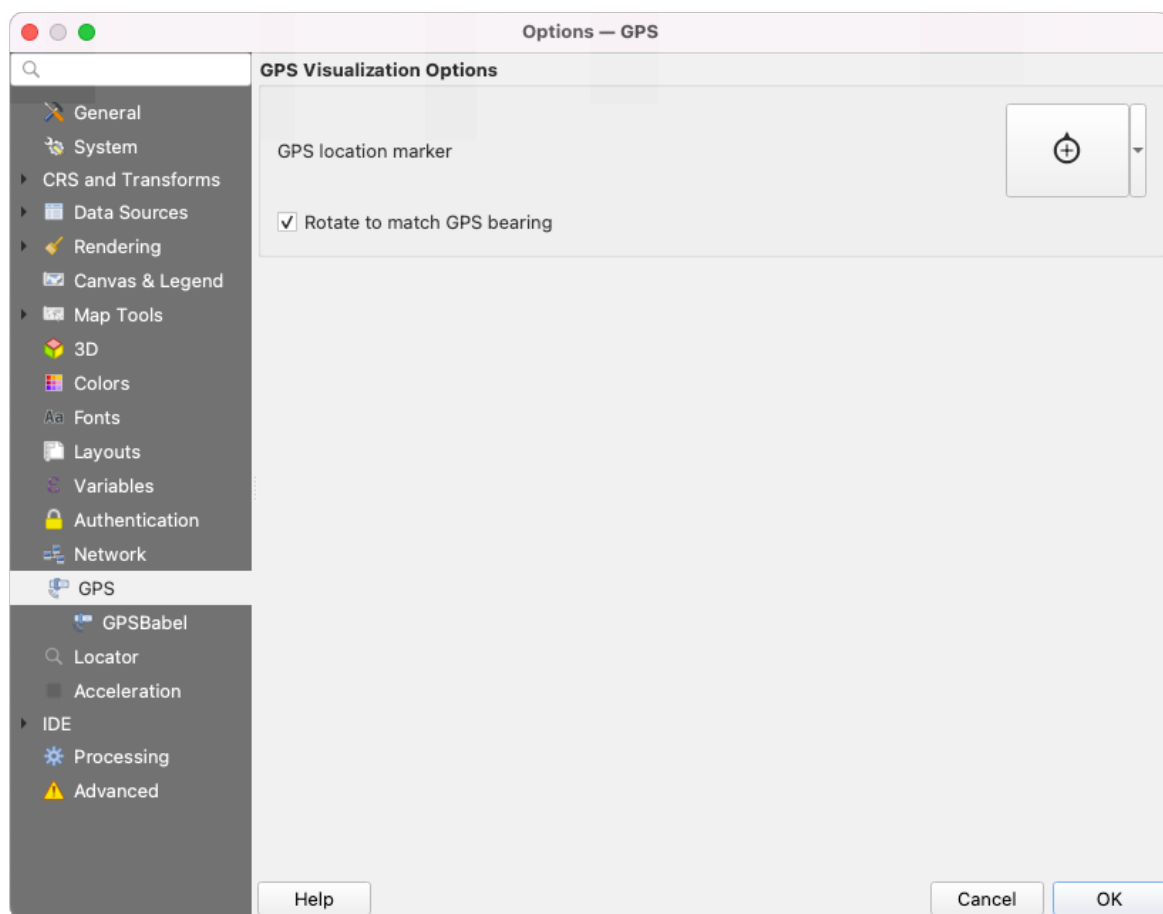
Fig. 9.23: Setări GPS
