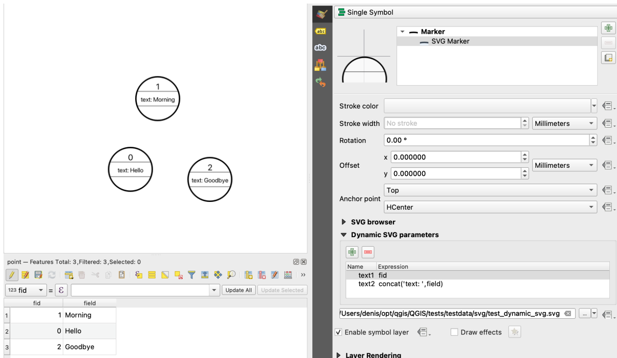
14.20. ábra: A Dinamikus SVG-paraméterek tábla
