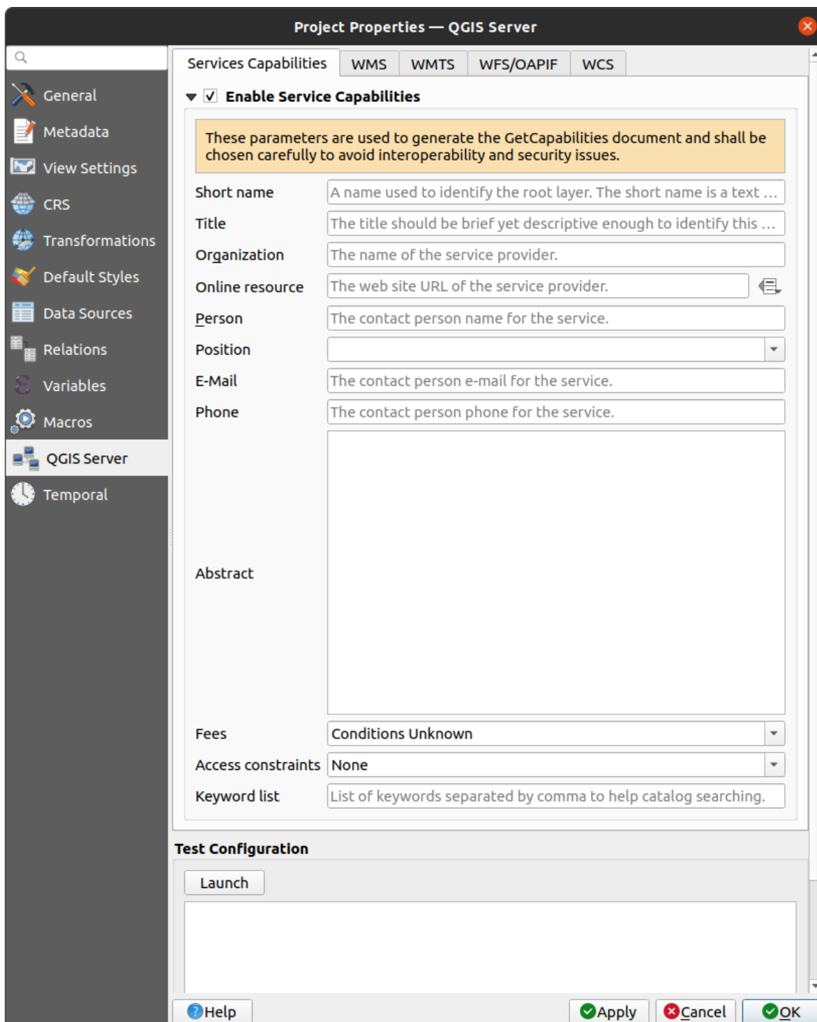
9.37. ábra: QGIS Server settings
