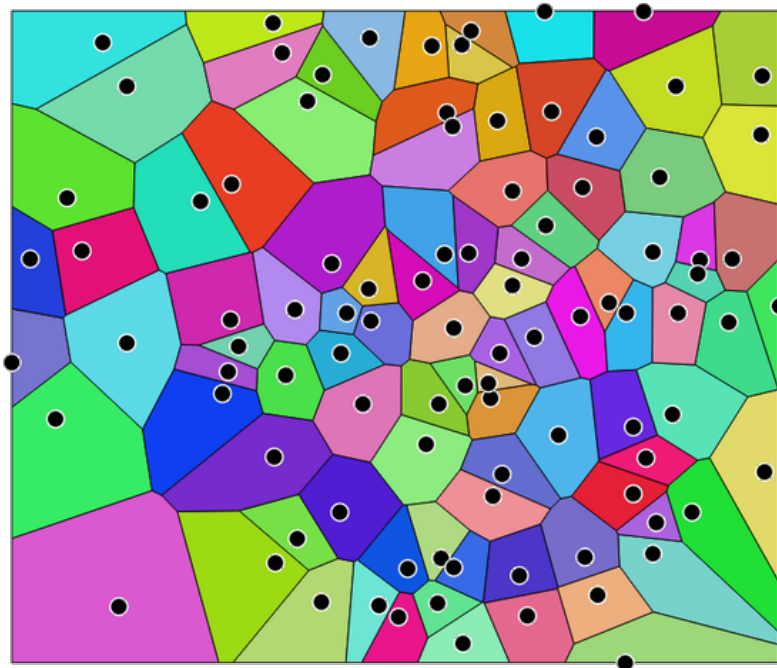
Fig. 27.108: Voronoi polygons
