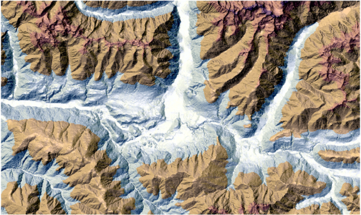
Fig. 27.26: Relief layer
