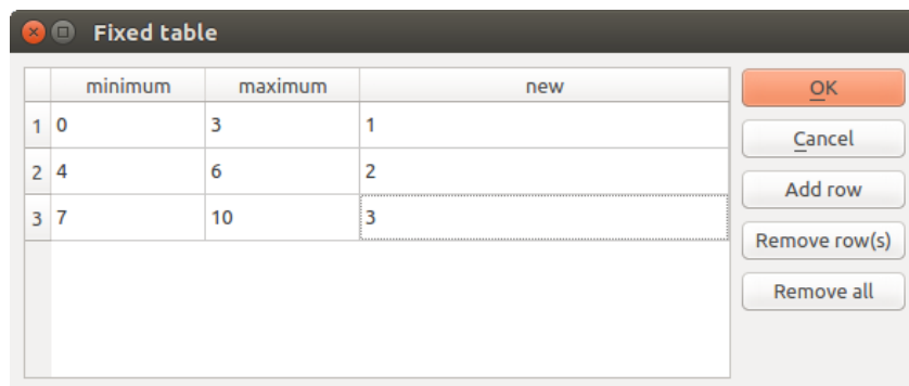
Fig. 26.14: Fixed Table
