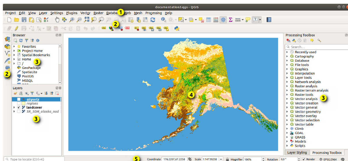
Fig. 11.1: QGIS GUI
