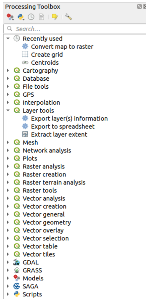
Obr. 26.6: Nástroje zpracování
