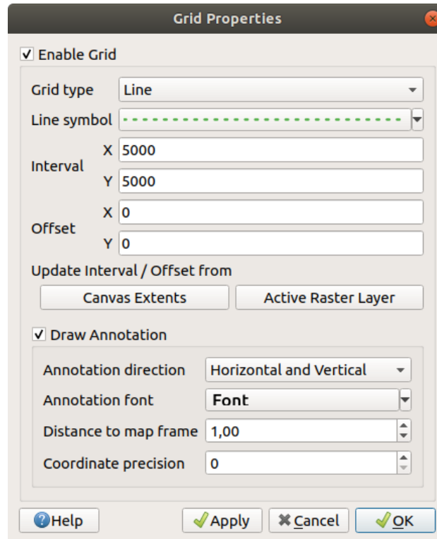
Obr. 11.5: Dialog mřížky
