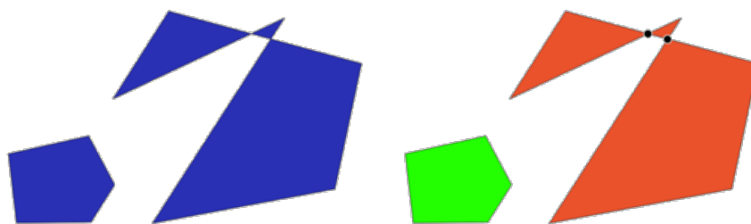
Рис. 25.57: Left: the input layer. Right: the valid layer (green), the invalid layer (orange)
