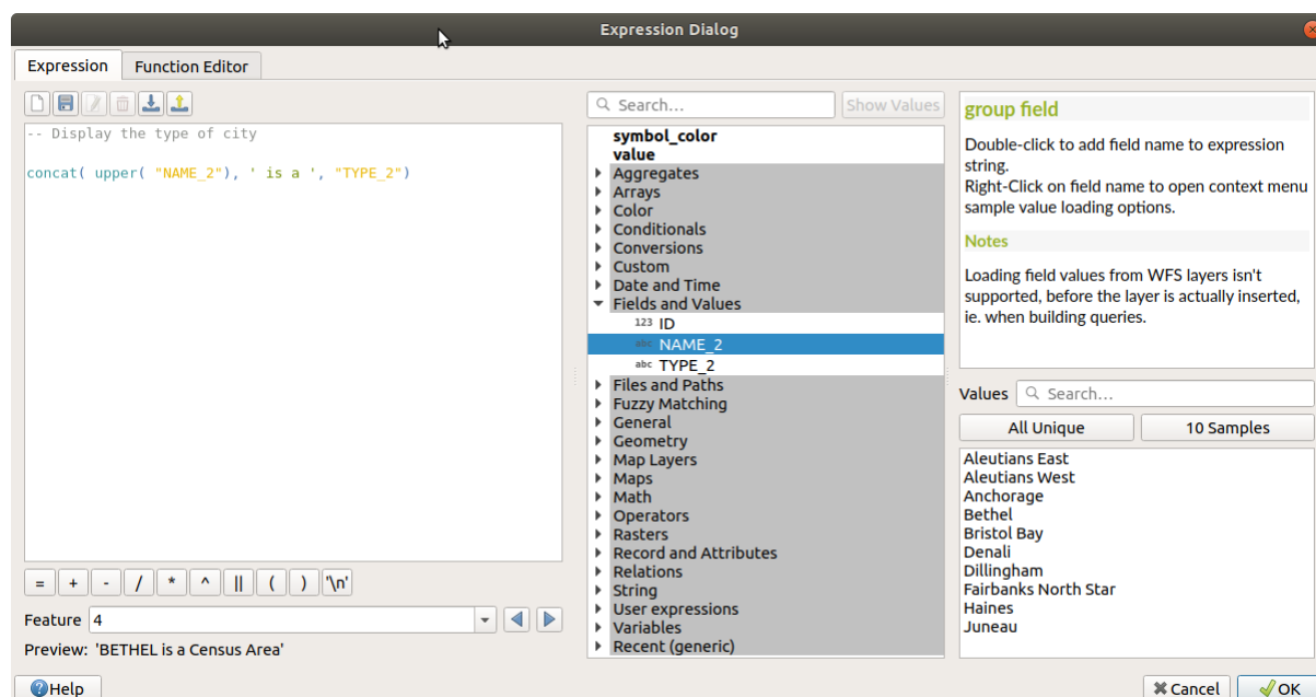
Рис. 12.1: The Expression tab
