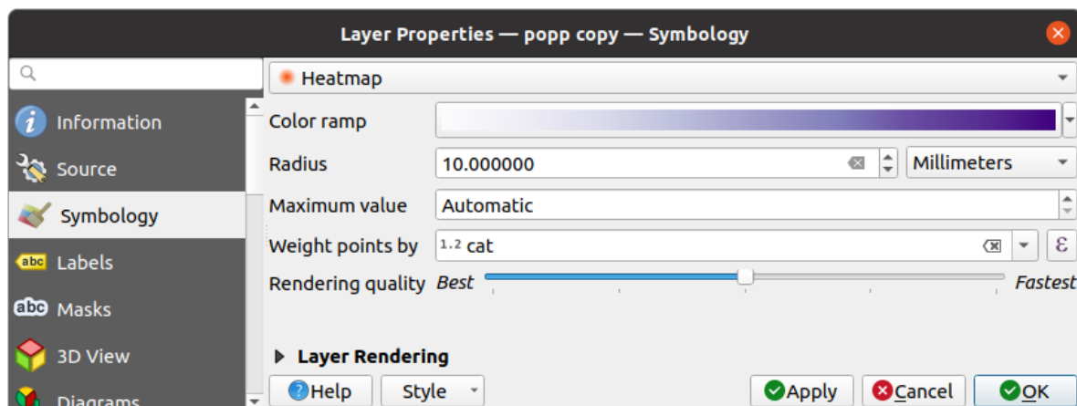
Рис. 15.11: Heatmap dialog
