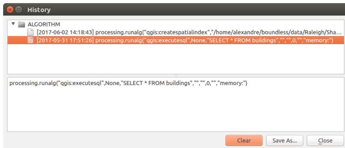
Рис. 24.15: History
