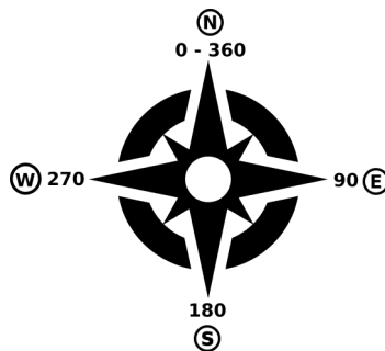
Рис. 25.21: Aspect values
