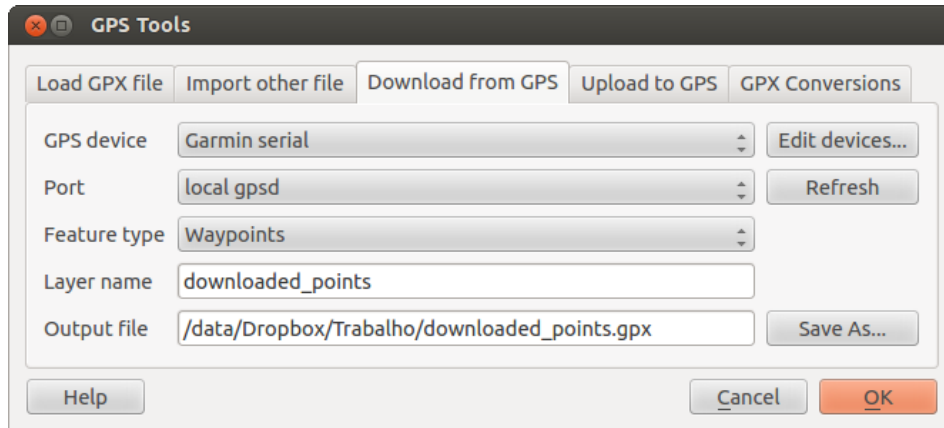
Рис. 21.2: Инструмент загрузки
