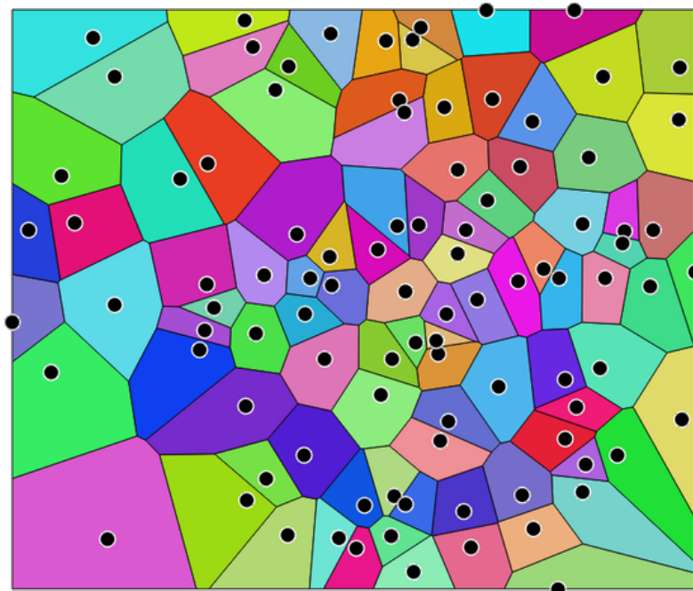
Рис. 25.100: Voronoi polygons
