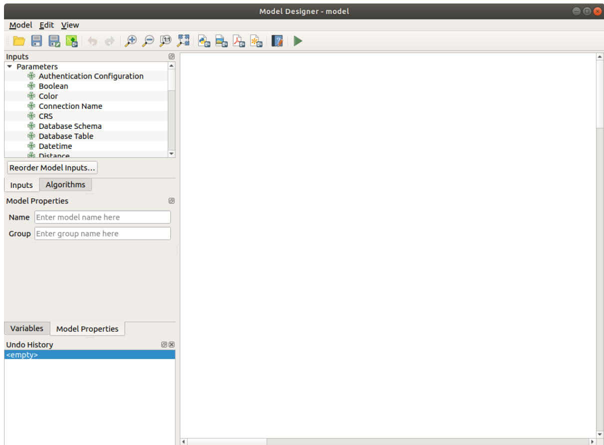
Рис. 24.16: Modeler
