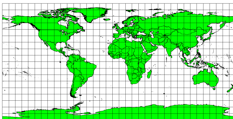
Figura 8.4: La proyección Plate Carree Cilíndrica Equidistante, por ejemplo, se utiliza cuando la precisión en la medida de distancias es importante.
