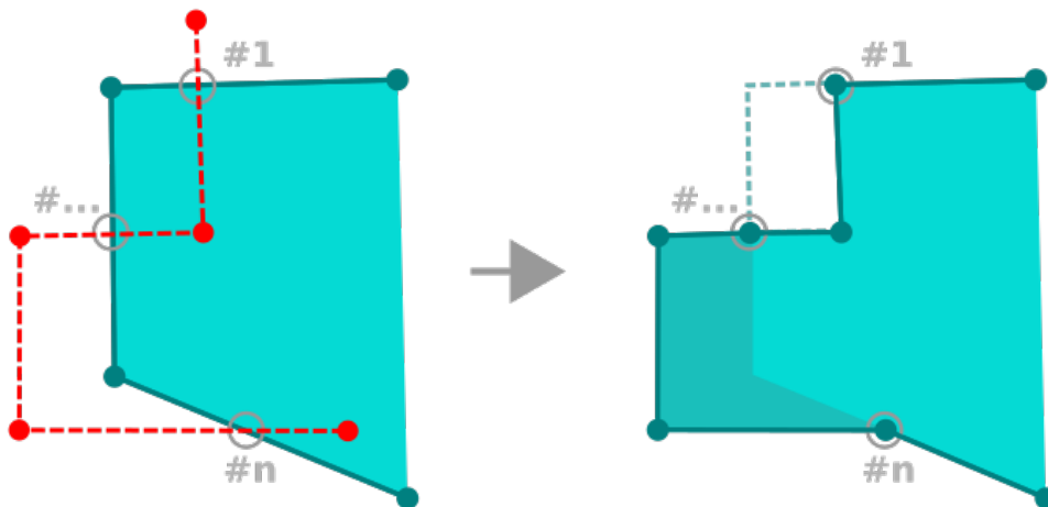
Şekil 14.92: Reshape polygon
