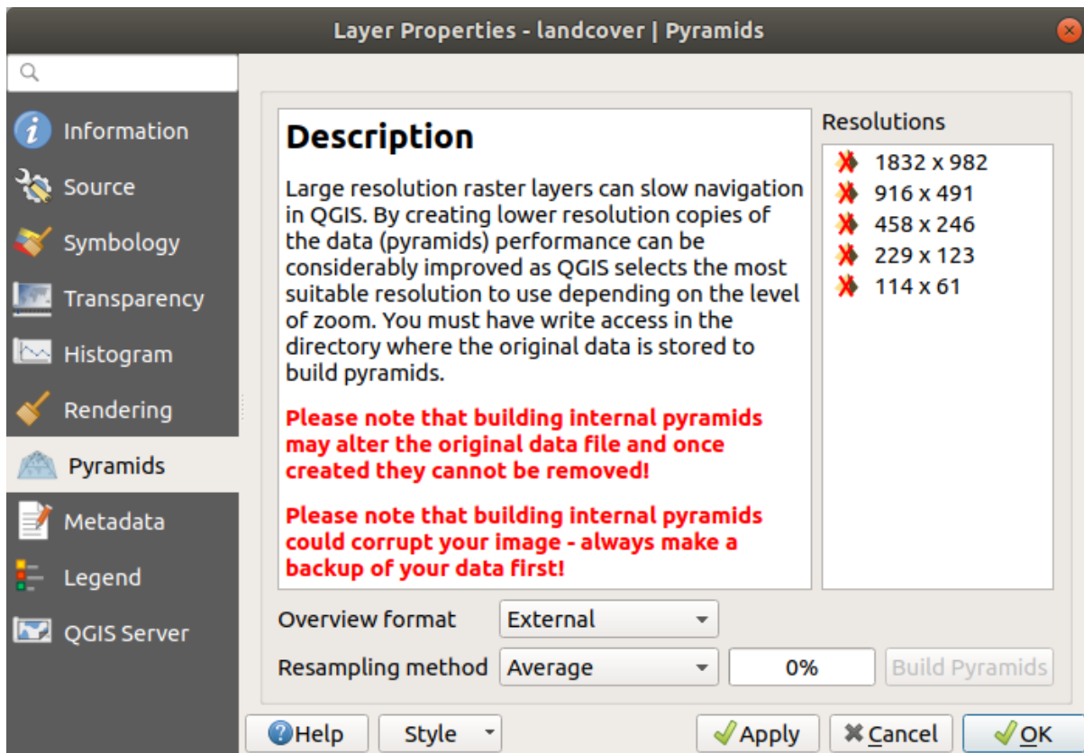
Şekil 15.13: Raster Pyramids
