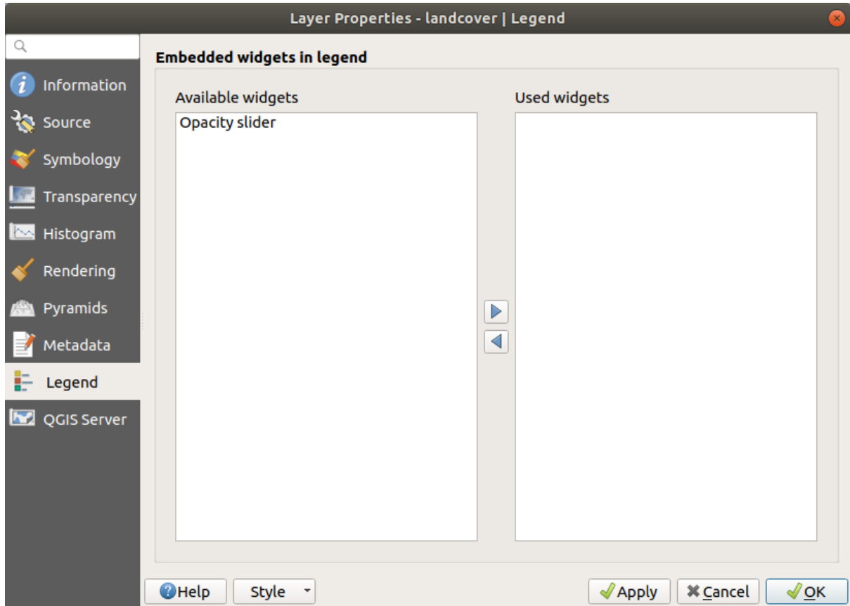
Şekil 15.15: Raster Legend
