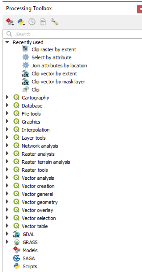
Şekil 23.1: Processing Toolbox
