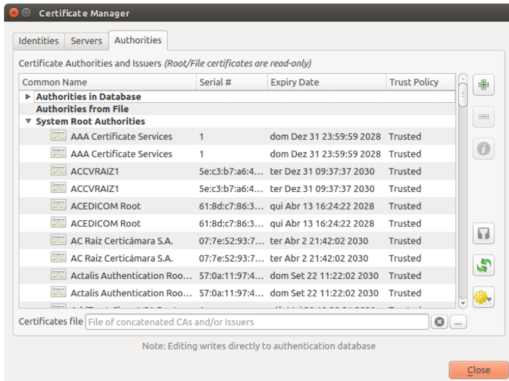
Şekil 21.24: Authorities editor
