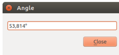
Şekil 11.19: Measure Angle
