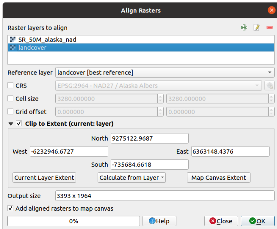
Şekil 15.19: Raster Alignment
