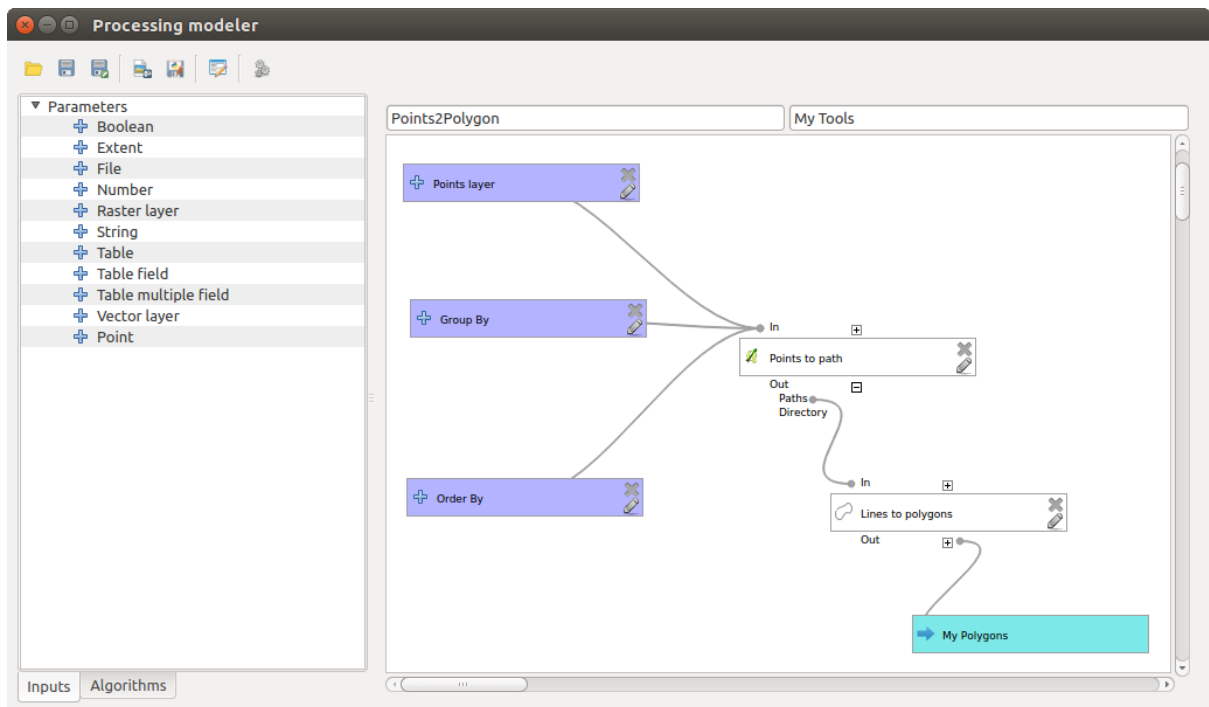
Şekil 23.2: Processing Modeler
