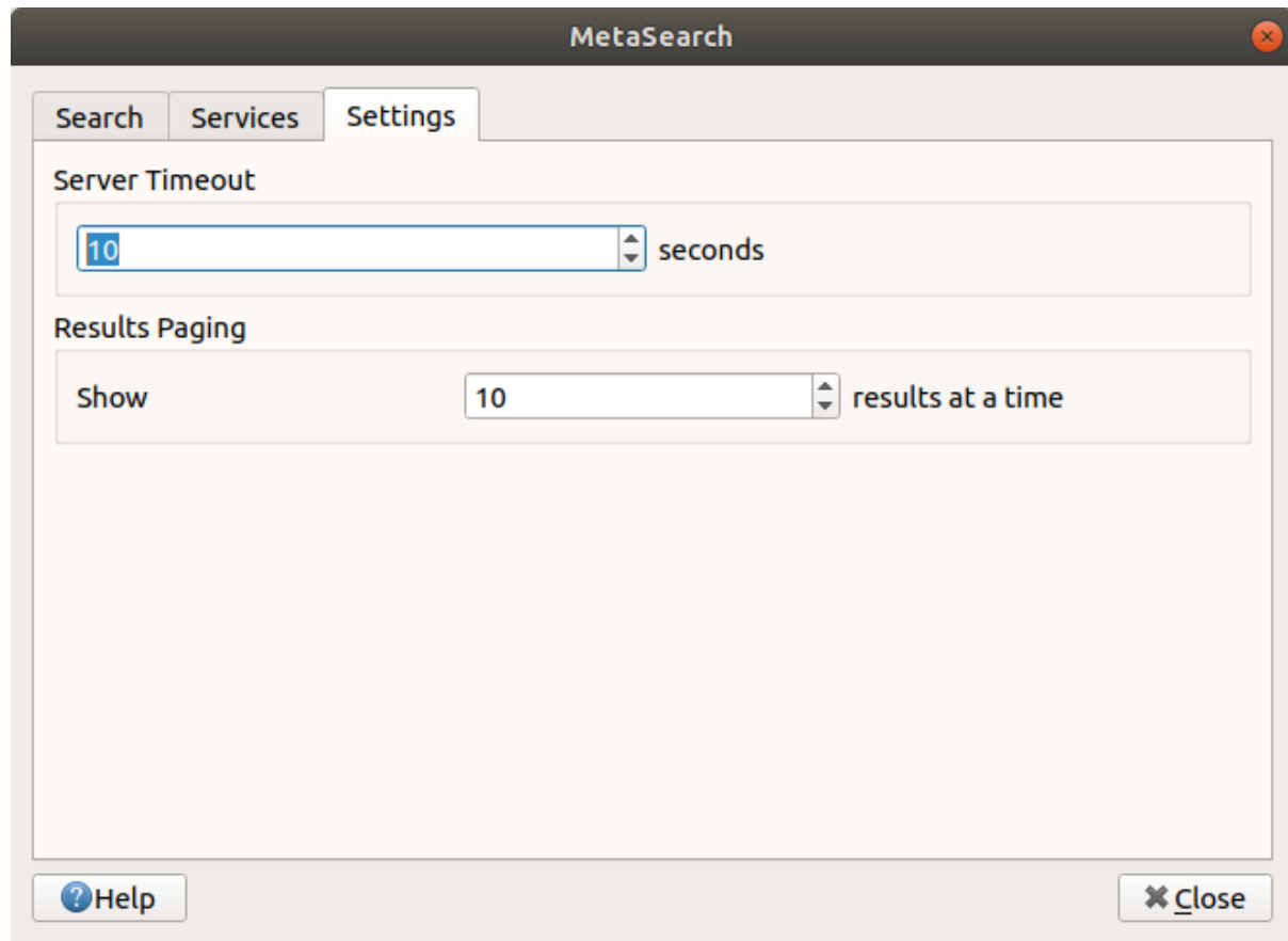
Şekil 25.16: MetaSearch settings
