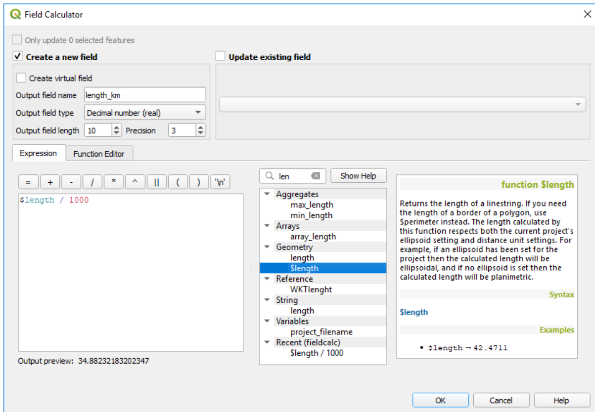
Şekil 14.73: Field Calculator
