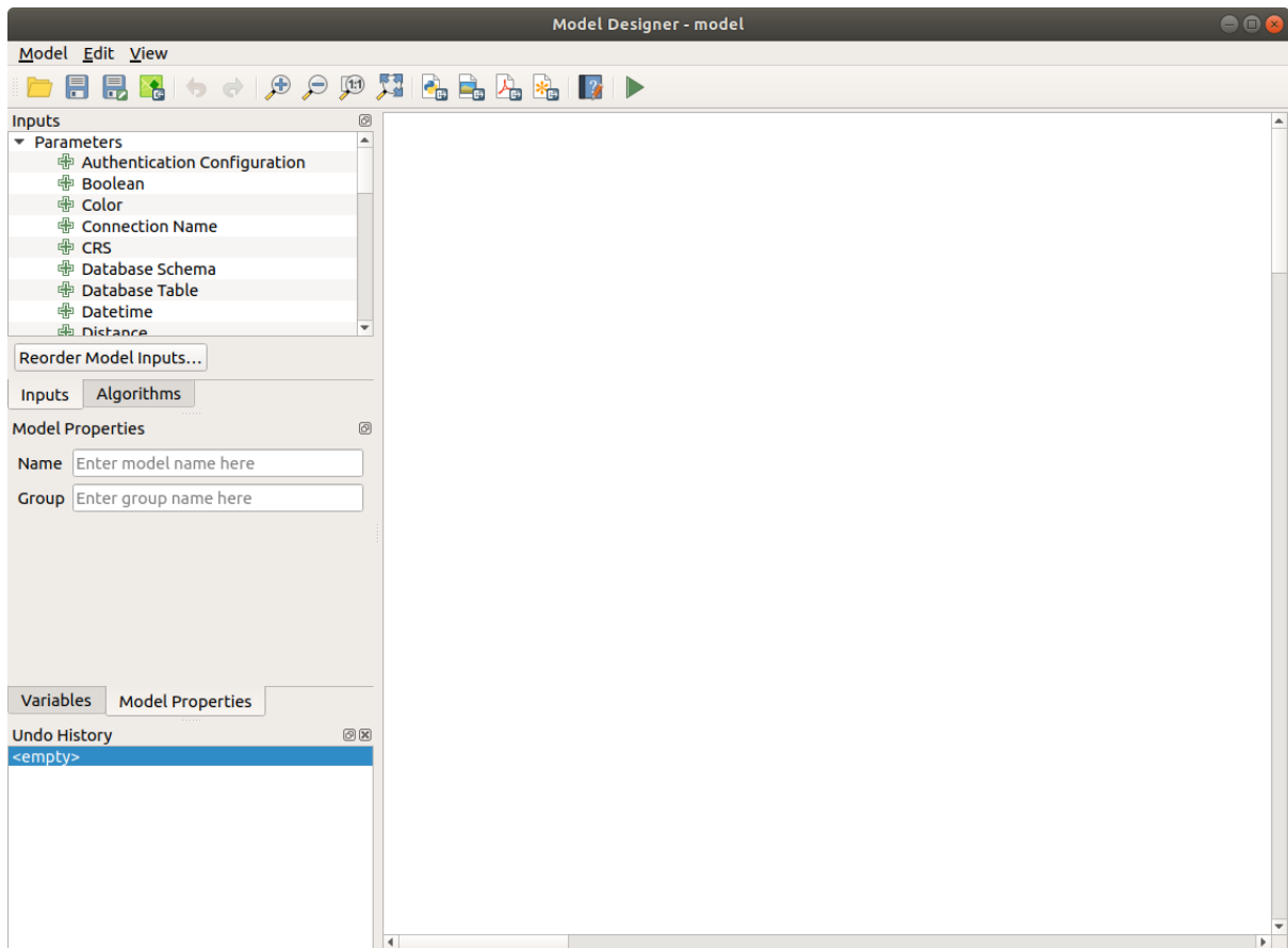
Şekil 23.16: Modeler
