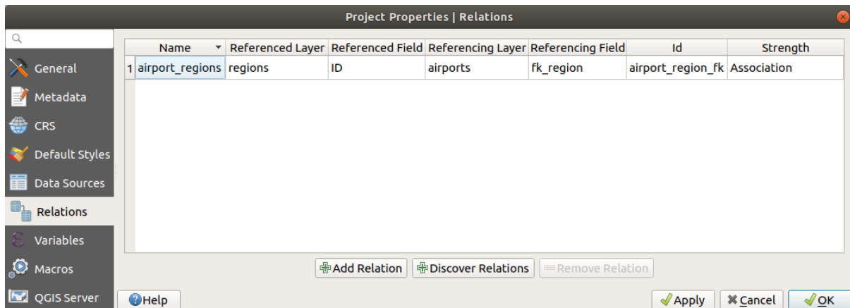
Şekil 9.26: Relations tab
