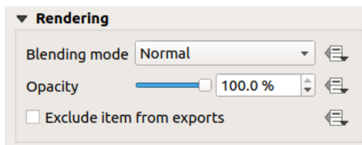
Şekil 18.13: Rendering mode
