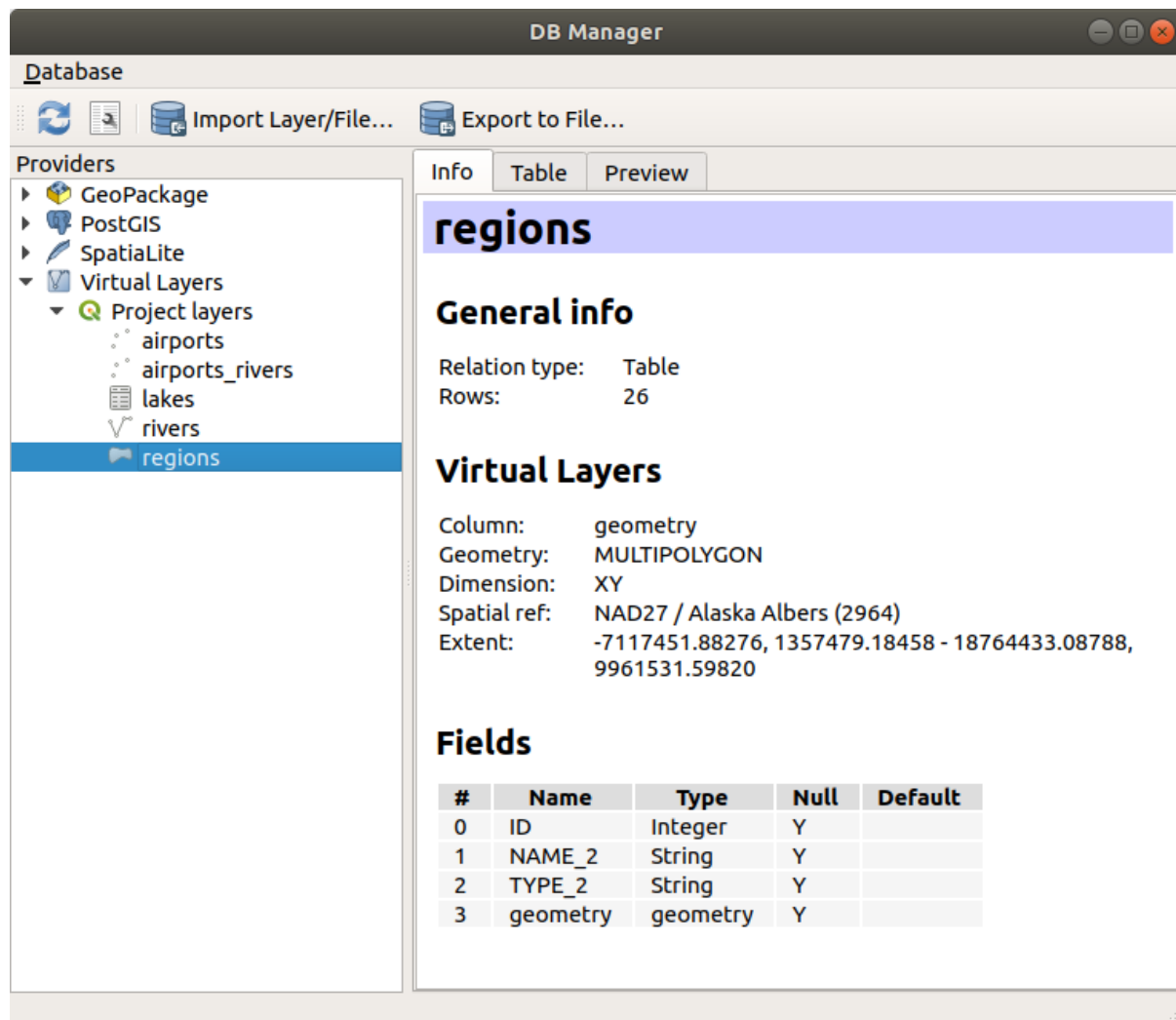
Şekil 25.8: DB Manager dialog
