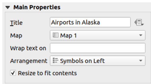
Şekil 18.26: Legend Main properties group
