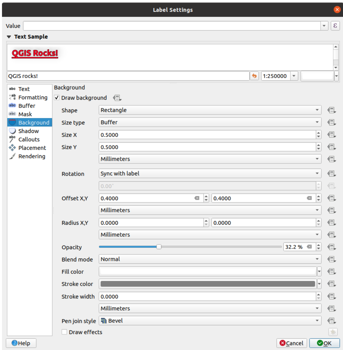
Şekil 12.18: Label settings - Background tab
