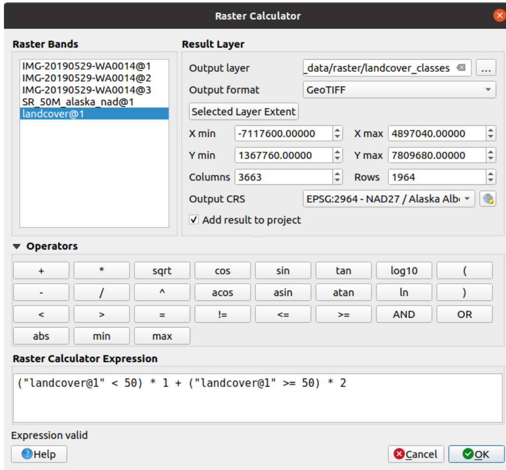
Şekil 15.17: Raster Calculator
