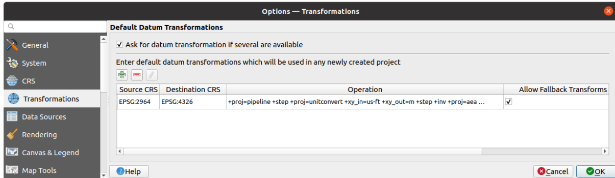
Şekil 9.3: Transformations Settings
