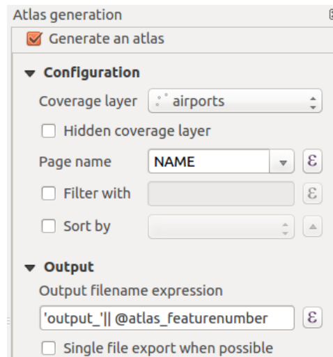
Şekil 18.62: Atlas Panel
