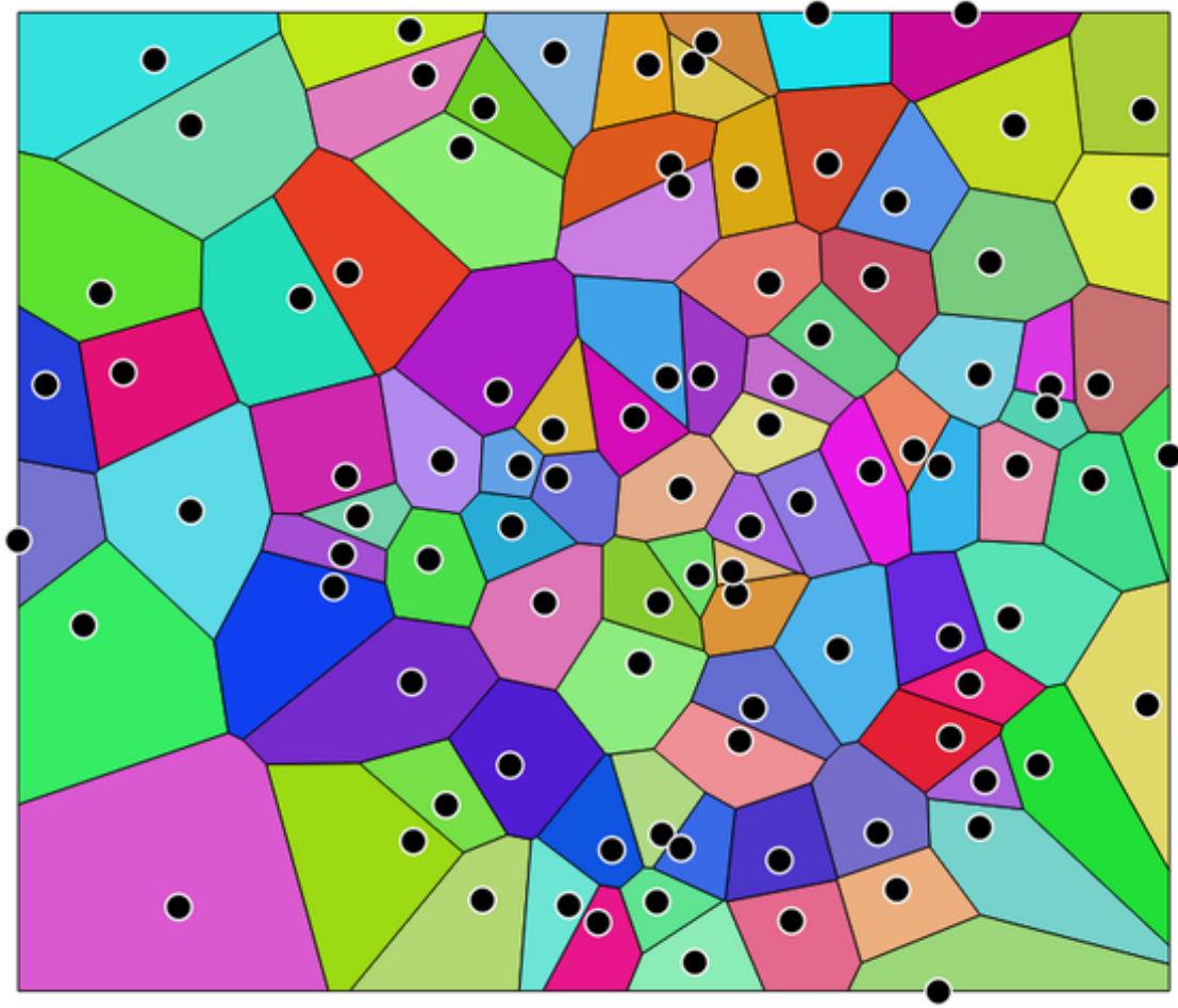
Şekil 24.91: Voronoi polygons
