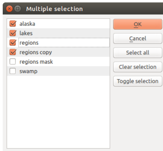
Şekil 23.12: Multiple Selection
