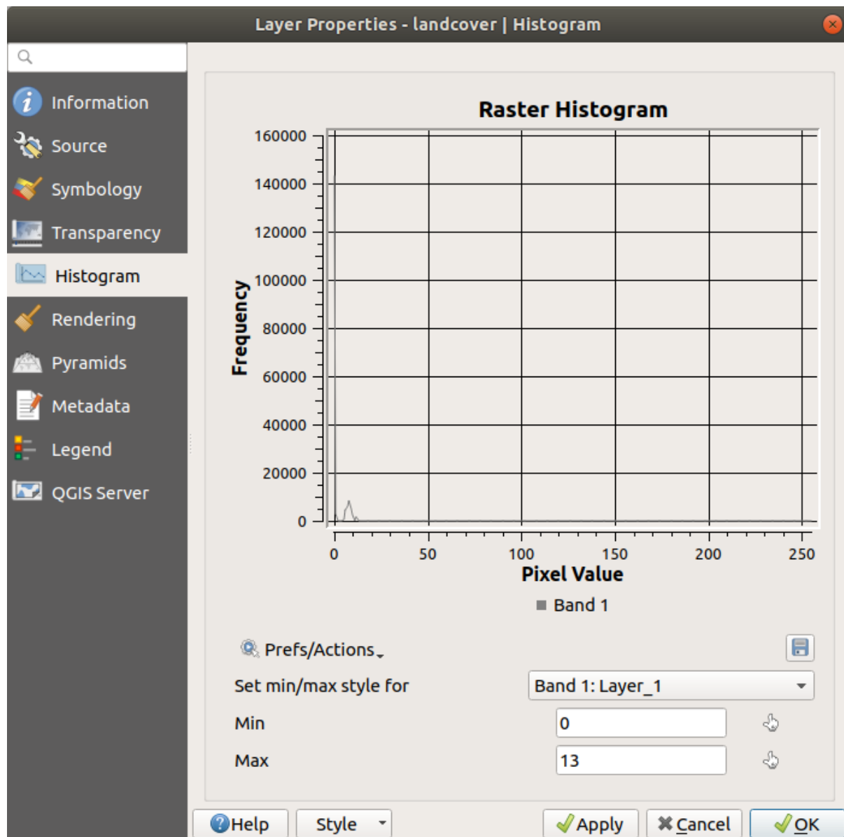
Şekil 15.11: Raster Histogram
