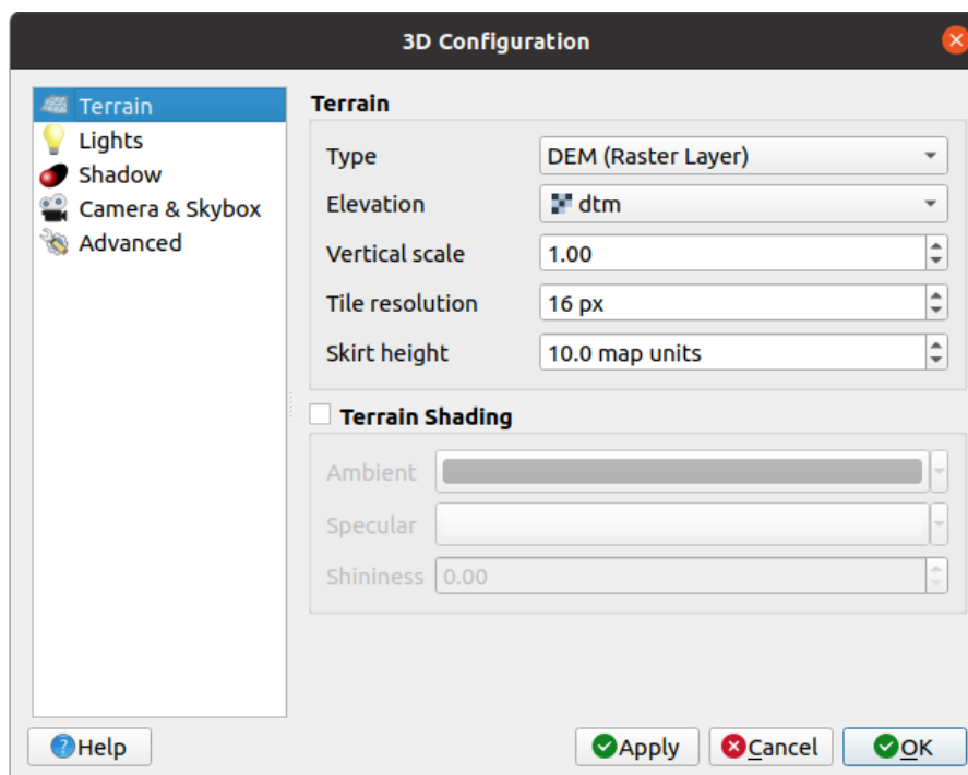
Şekil 7.8: The 3D Map Configuration dialog
