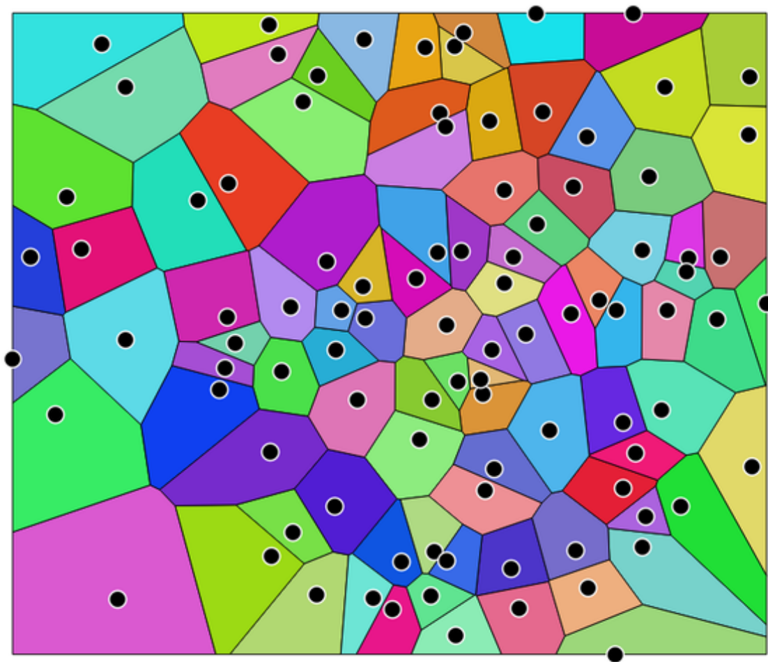
Рис. 24.91: Voronoi polygons
