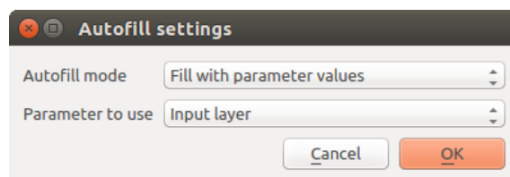
Рис. 23.32: Диалог автозаполнения
