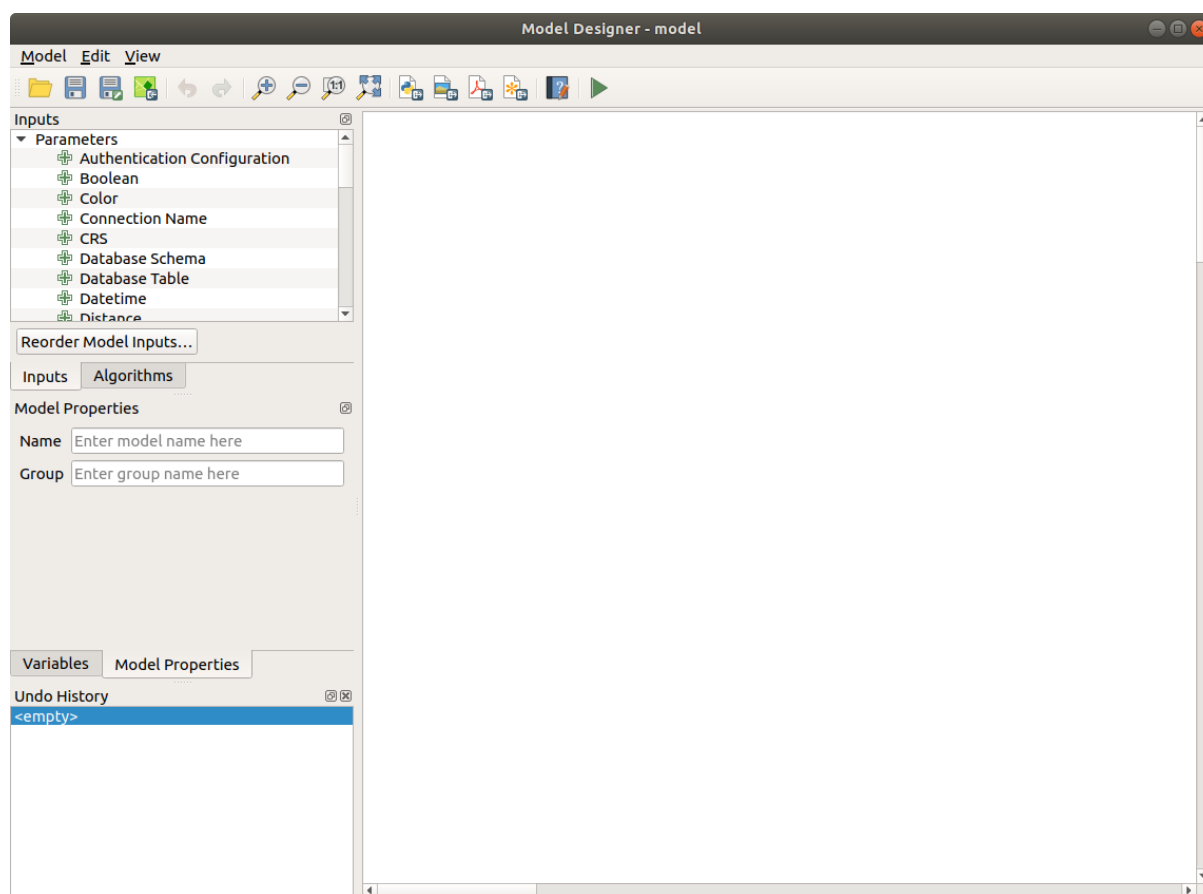
Рис. 23.16: Modeler
