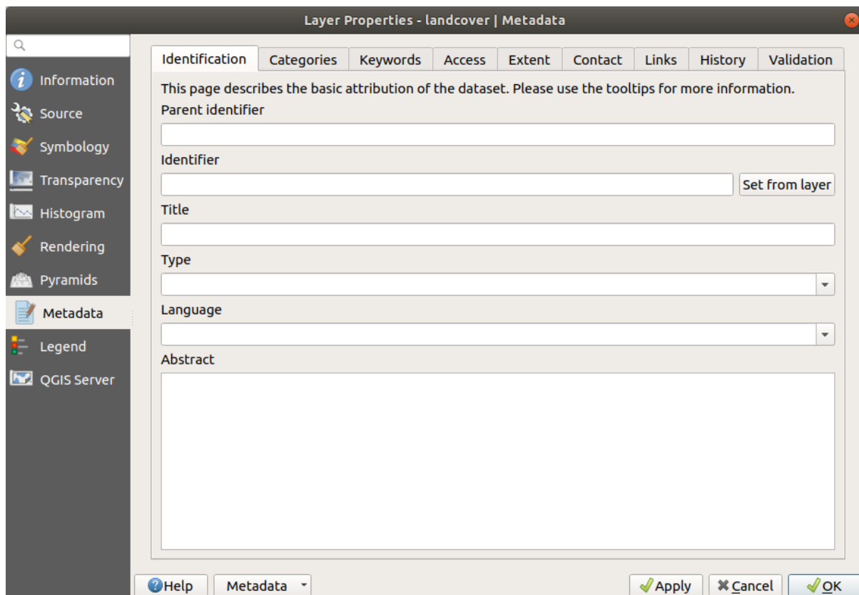
Рис. 15.14: Raster Metadata
