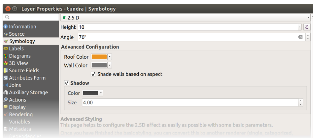
Рис. 14.13: 2.5D dialog
