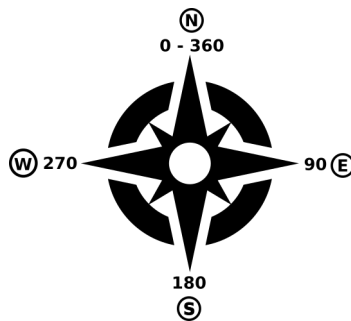
Gambar24.16: Aspect values
