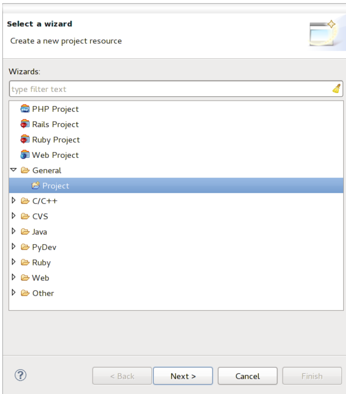
图 16.1: Eclipse project
