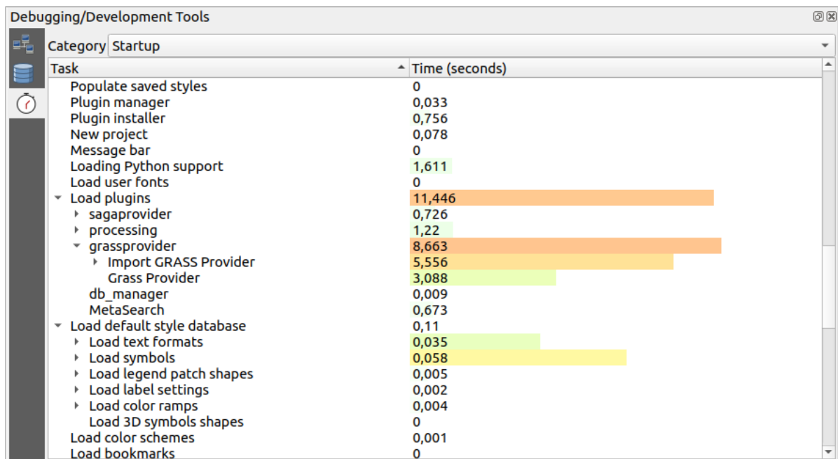
図 12.8: QGIS の起動に関するプロファイル
