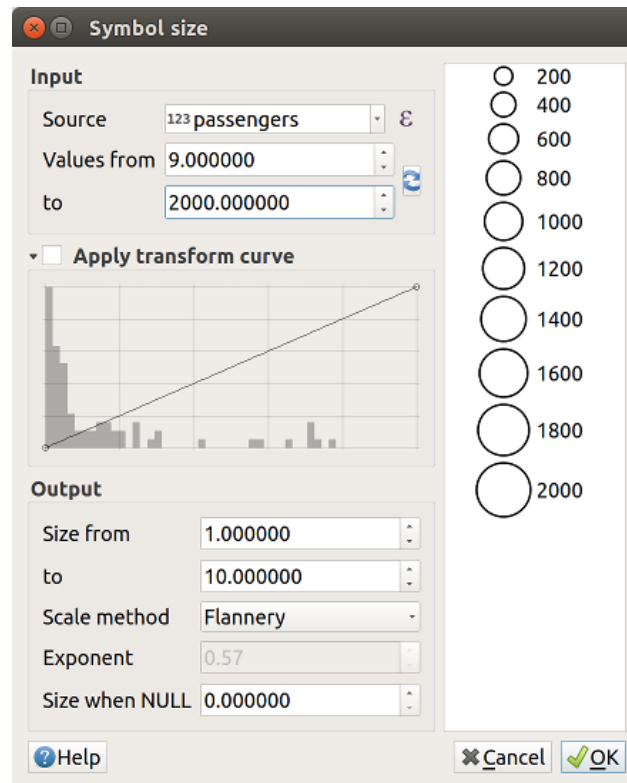
図 12.29: passengers レイアのフィールド値に基づいた地物サイズのスケーリング
