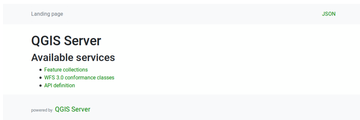
Fig. 3.24: Server OAPIF startpagina
