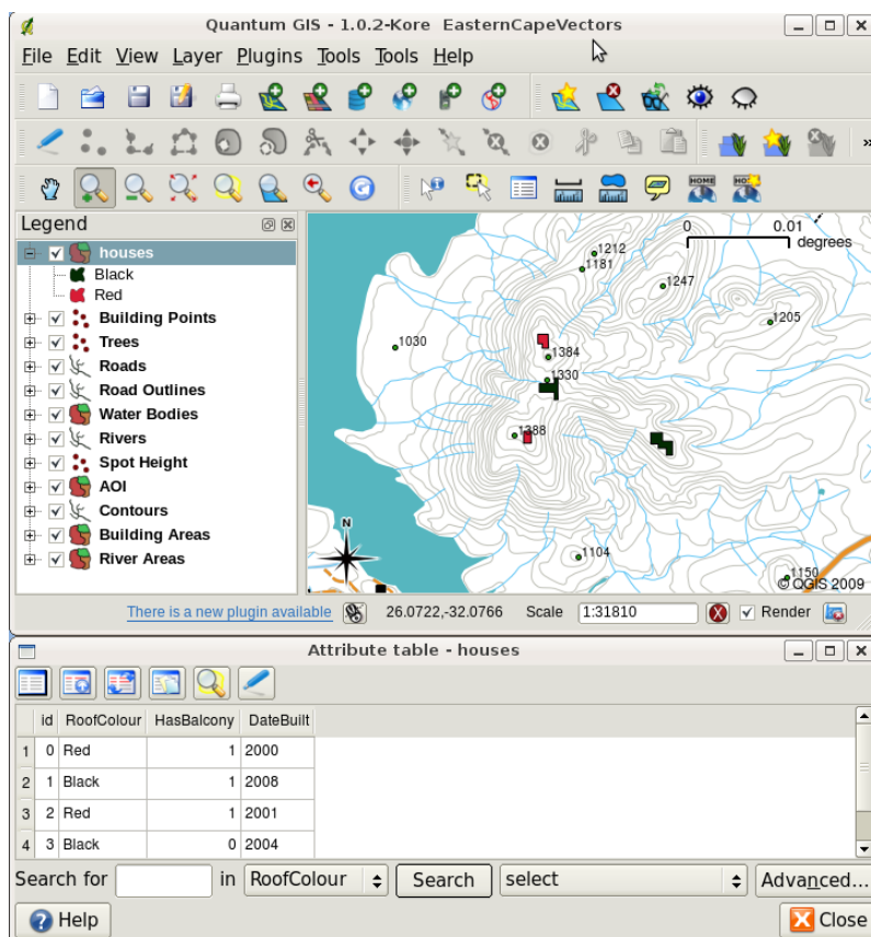
図 4.3: 家のレイヤ。家の地物には、屋根の色等の属性やその他属性情報が記述されています。属性テーブル(下図)には、地図上に示された家エリアの属性のリストが示されています。テーブルの中で地物が強調表示されているときは、地図上では黄色のポリゴンとして見えます。
