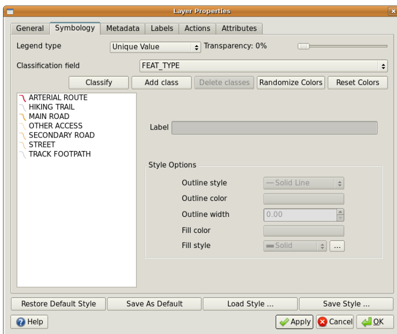
図 4.13: 道路の種類に基づいて、道路に対して一意値シンボルを定義します。
