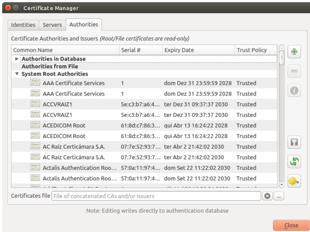
Fig. 25.24: Editor Autorità
