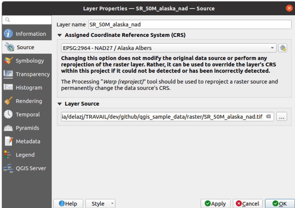
Figura 17.1: Propiedades de capa Ráster - Diálogo Fuente
