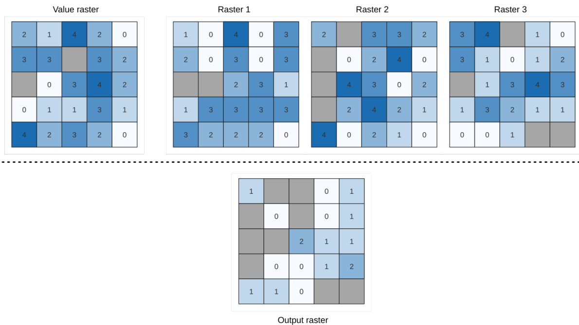
Figura 28.22: Para cada celda del ráster de salida, el valor representa la cantidad de veces que las celdas correspondientes en la lista de rásteres son iguales al ráster de valores. Se tienen en cuenta las celdas sin datos (grises).
