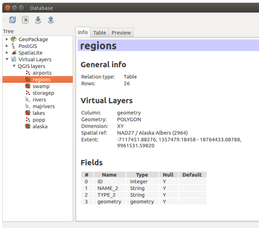
Фигура 11.2: DB Manager dialog
