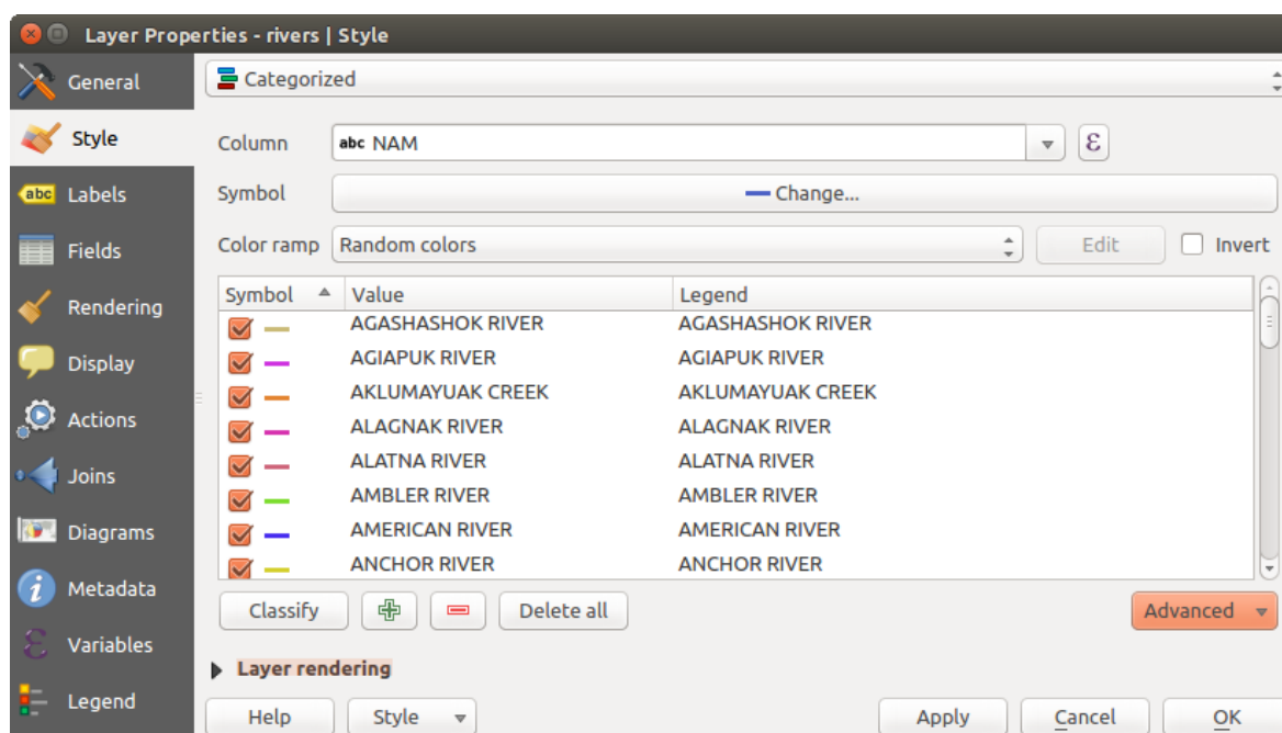
Фигура 12.10: Categorized Symbolizing options
