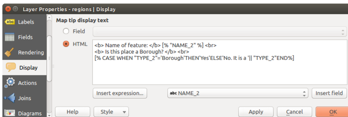
Фигура 12.52: HTML code for map tip
