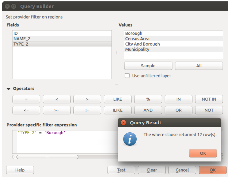
Фигура 12.8: Query Builder
