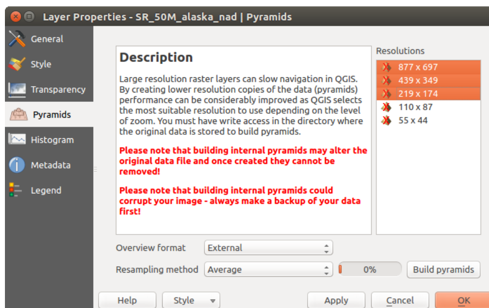
Фигура 13.7: Raster Pyramids
