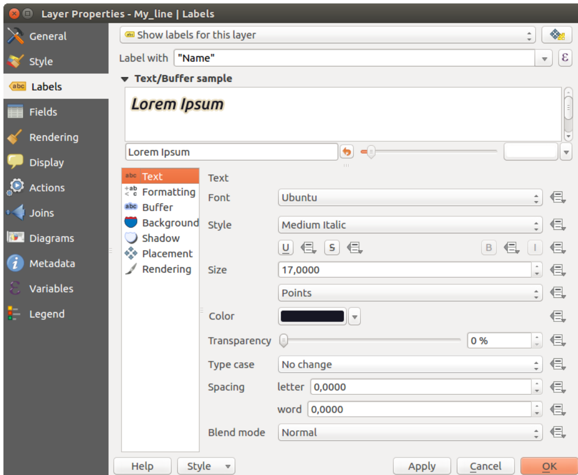
Фигура 12.30: Layer labeling settings - Text tab
