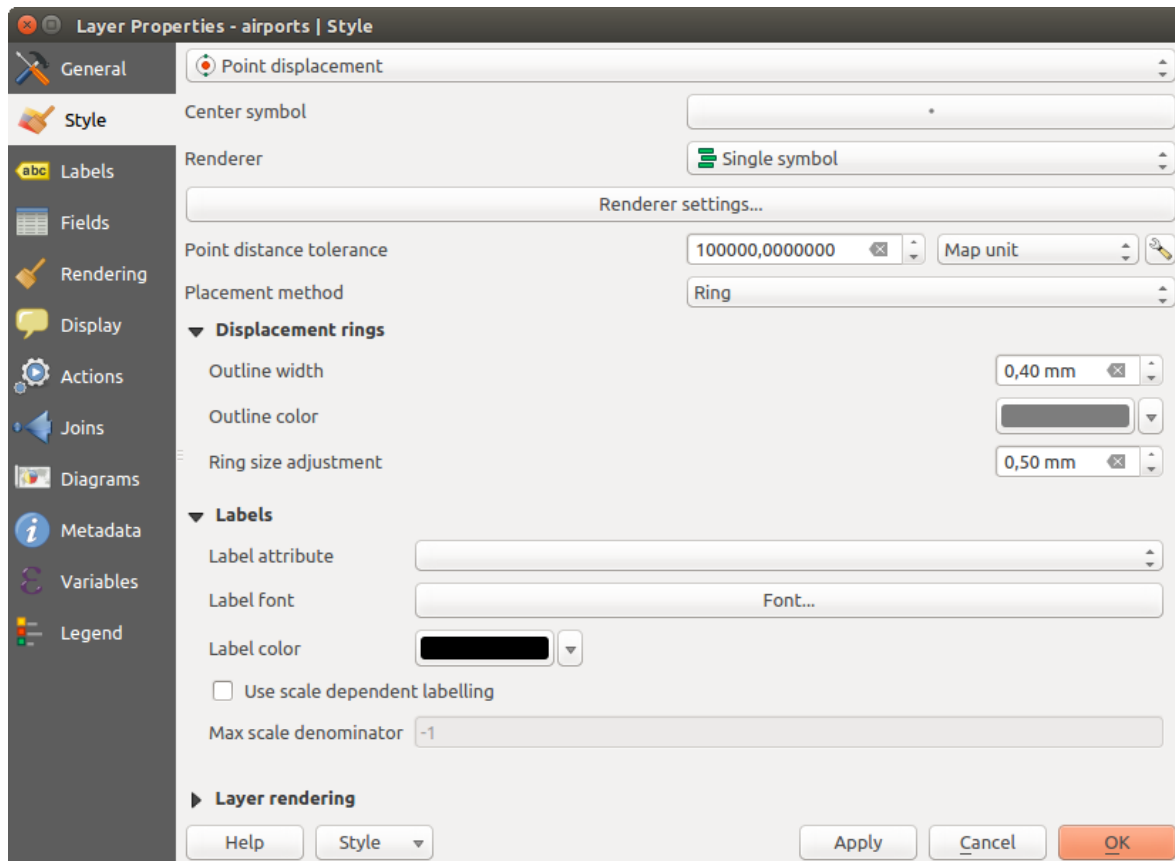
Фигура 12.15: Point displacement dialog
