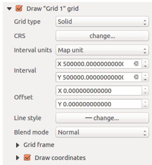
Фигура 14.15: Draw Grid Dialog
