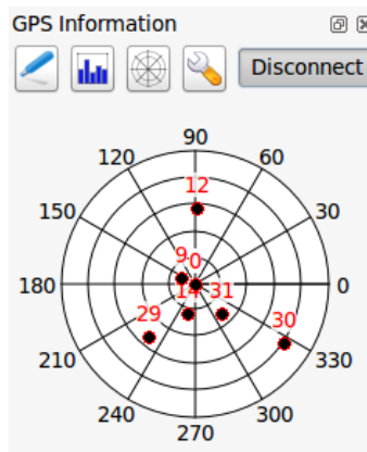
Фигура 16.5: GPS tracking polar window
