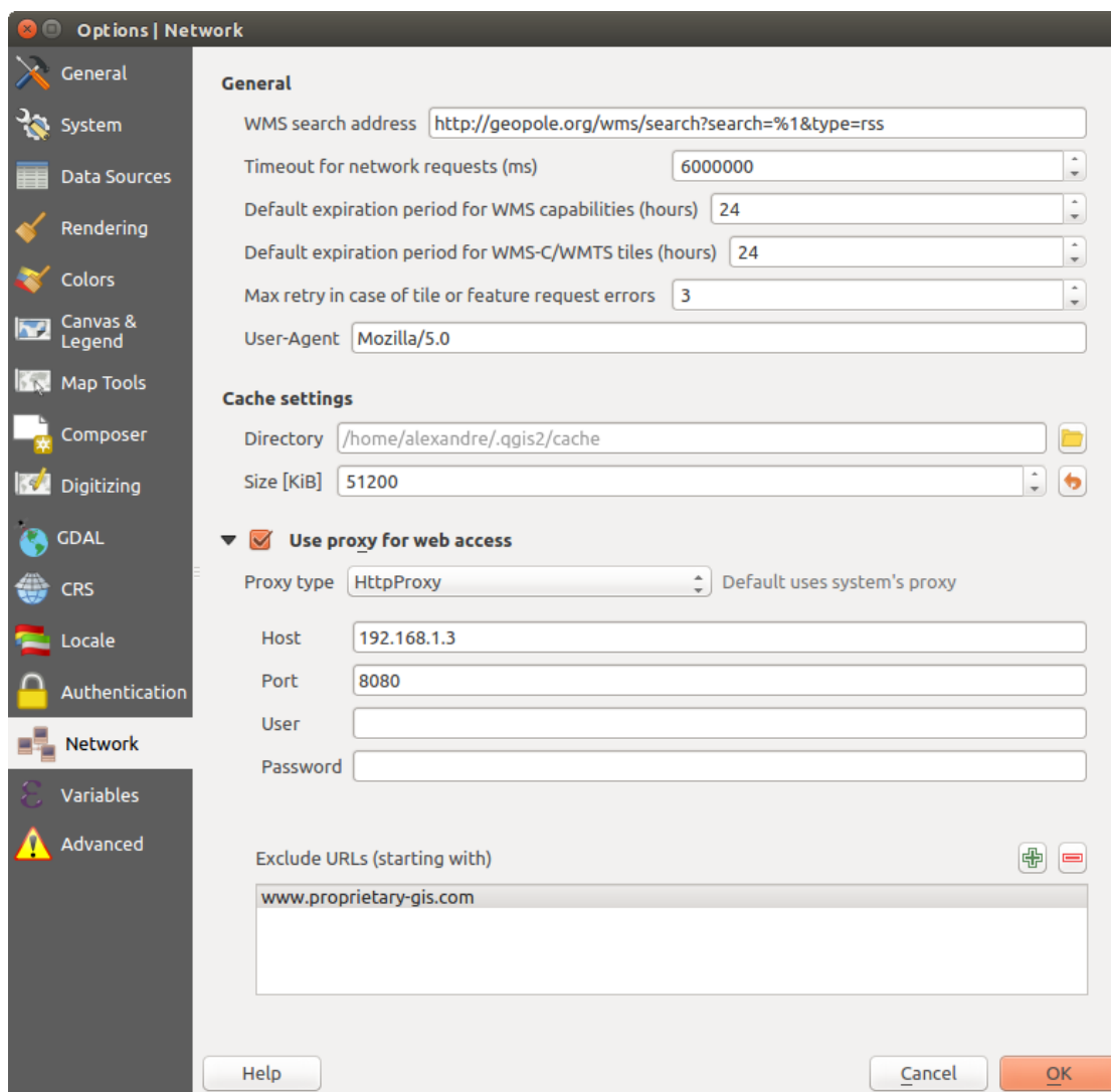
Фигура 9.3: Proxy-settings in QGIS
