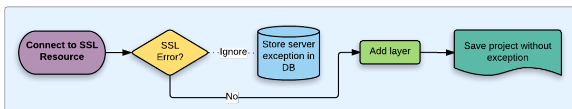
Фигура 17.33: SSL server exception
