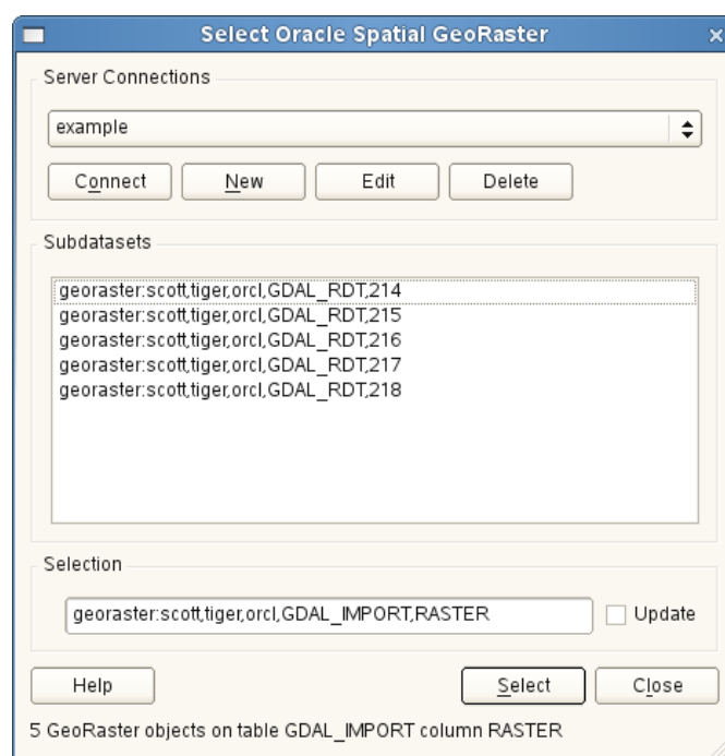
Фигура 21.38: Select Oracle GeoRaster dialog
