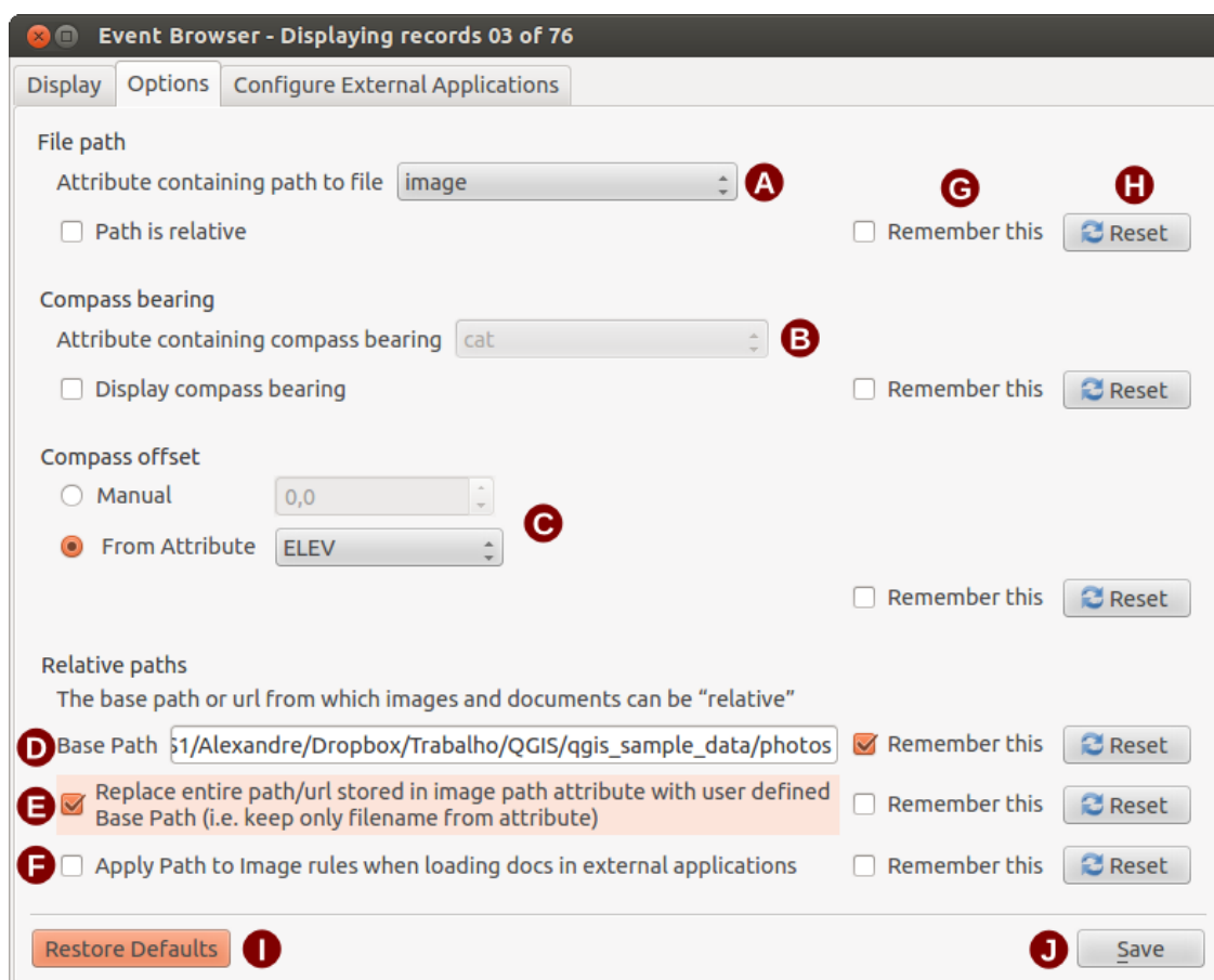
Фигура 21.14: The eVis Options window
