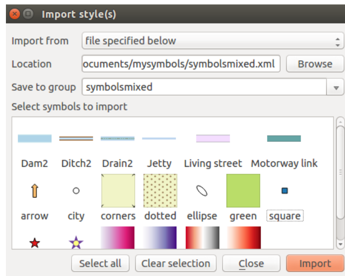
Фигура 12.3: Importing symbols
