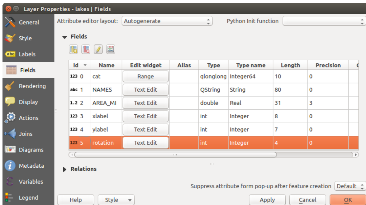
Фигура 12.39: Field properties tab
