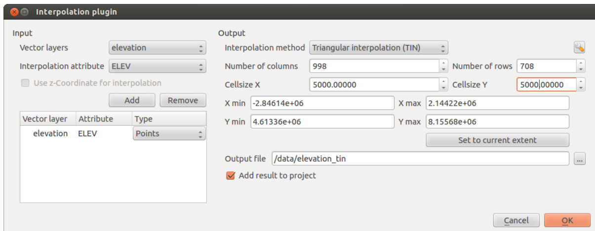
Фигура 21.30: Interpolation Plugin
