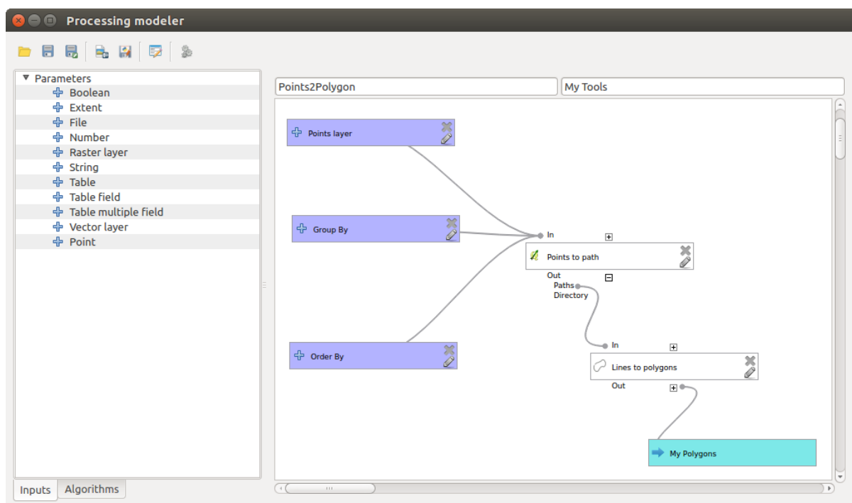
Фигура 20.2: Processing Modeler
