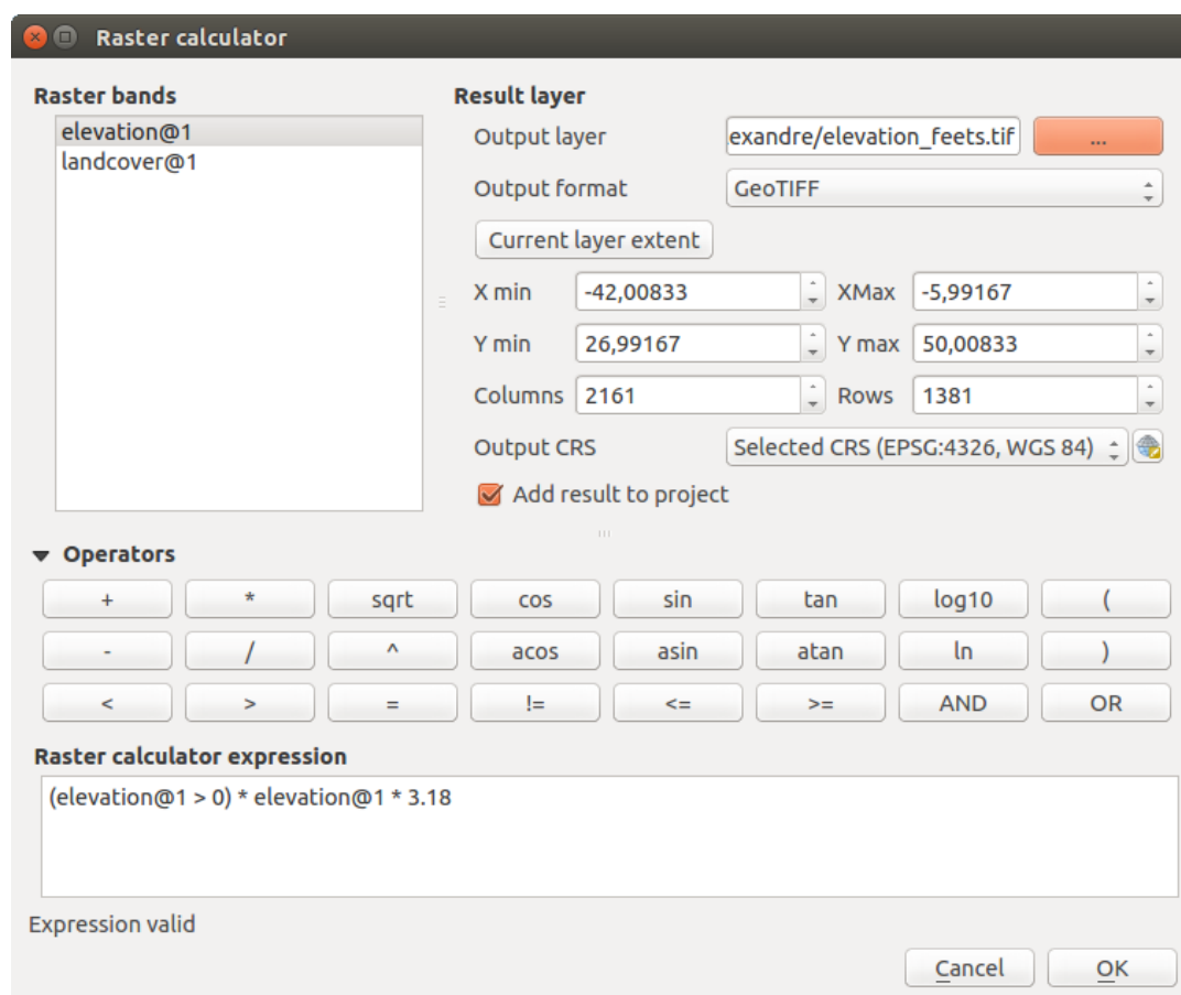
Фигура 13.10: Raster Calculator
