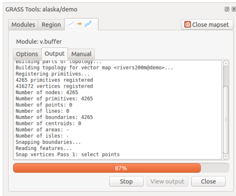
Фигура 18.5: GRASS Toolbox Module Output
