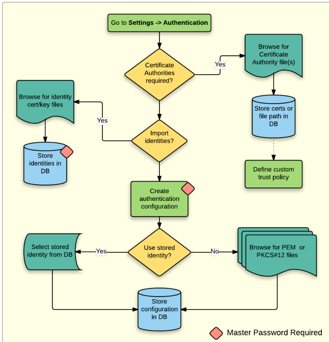
Фигура 17.20: PKI configuration workflow
