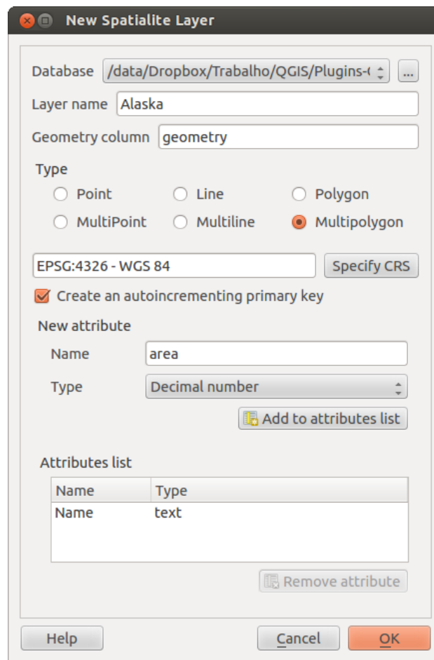
Фигура 11.10: Creating a New Spatialite layer dialog
