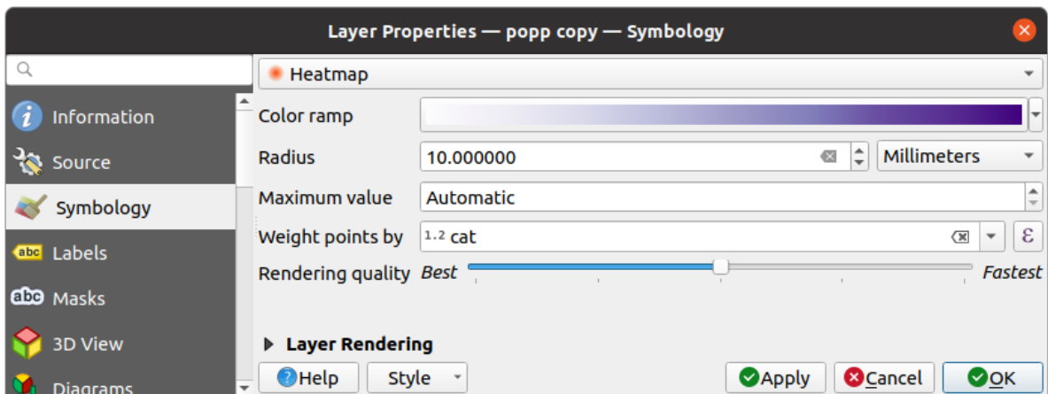
Рис. 16.11: Heatmap dialog
