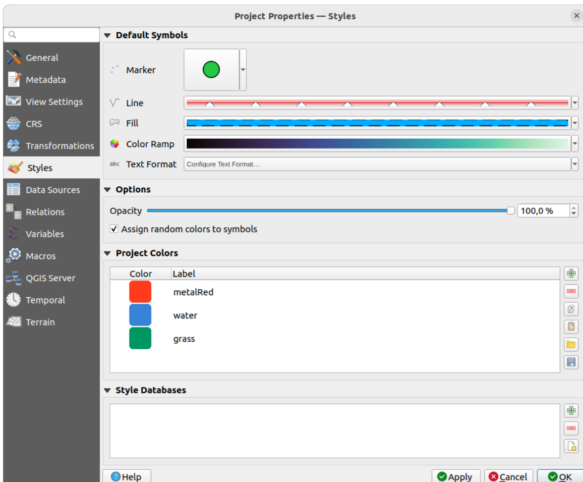
Рис. 9.34: Styles tab
