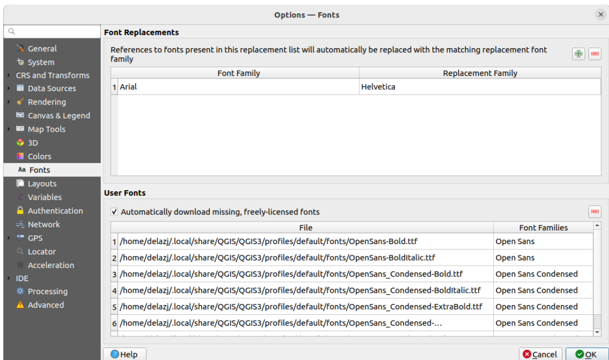
Рис. 9.19: Fonts settings
