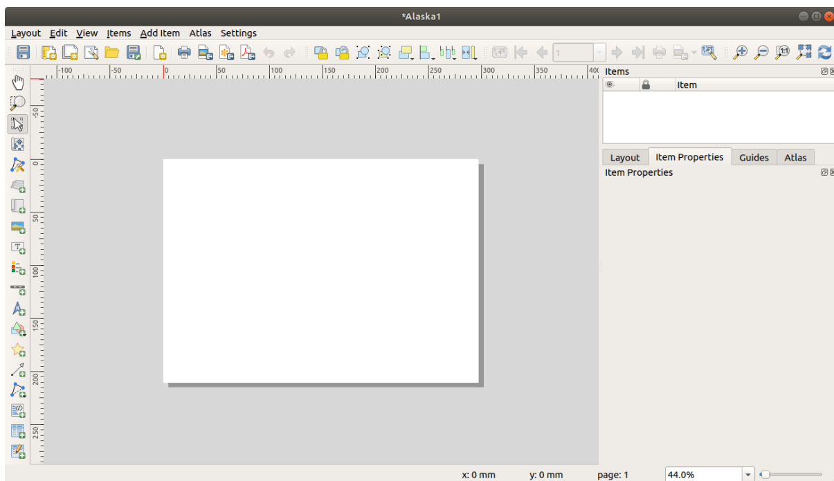
Рис. 22.2: Print Layout
