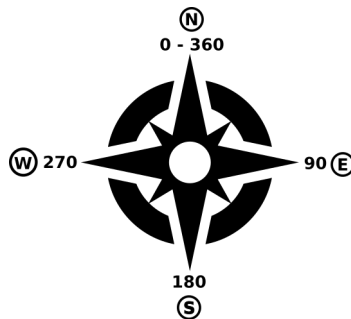
Figura28.29: Gama de valores da Exposição
