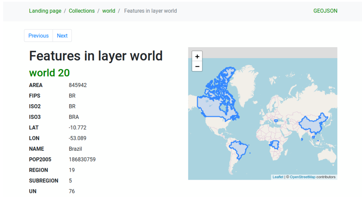
그림 3.27: 서버 OAPIF 피처 목록 페이지
