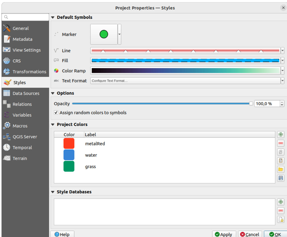
Obr. 9.34: Styles tab
