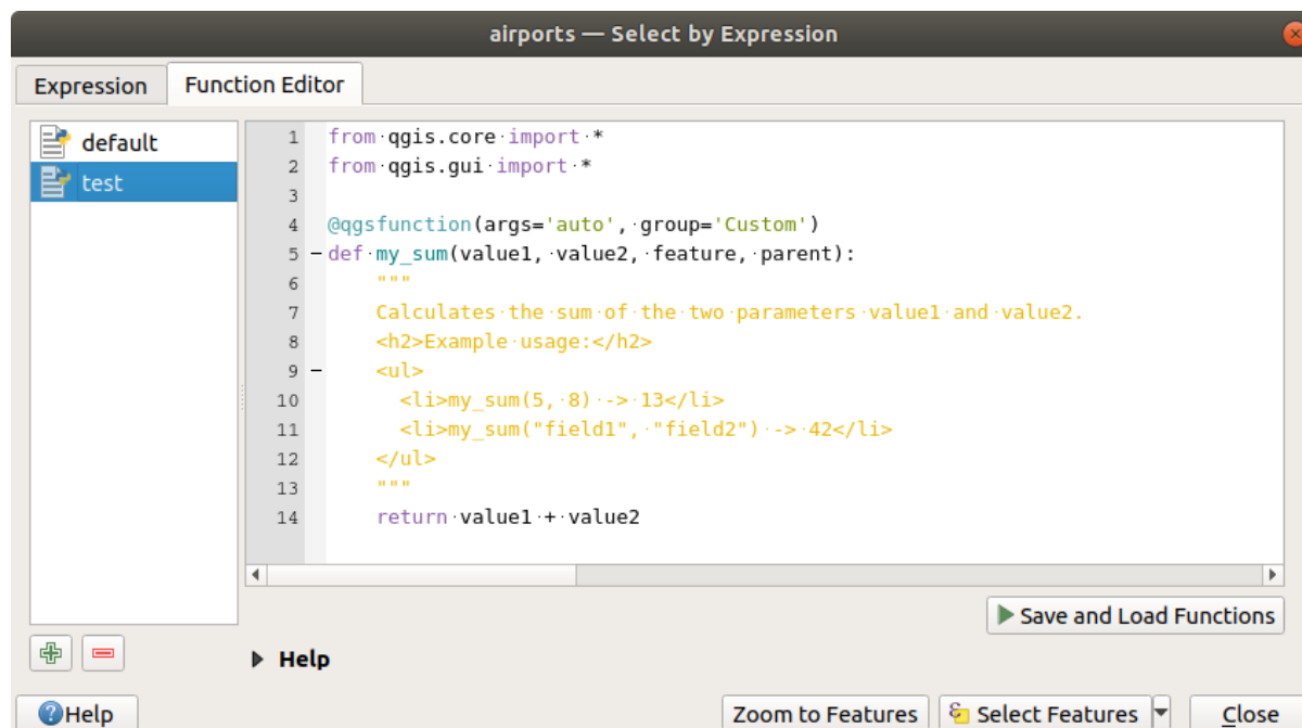
Рис. 13.2: The Function Editor tab
