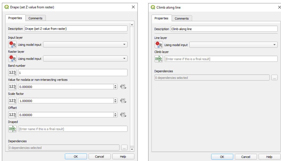
Рис. 27.22: Model Algorithm parameters
