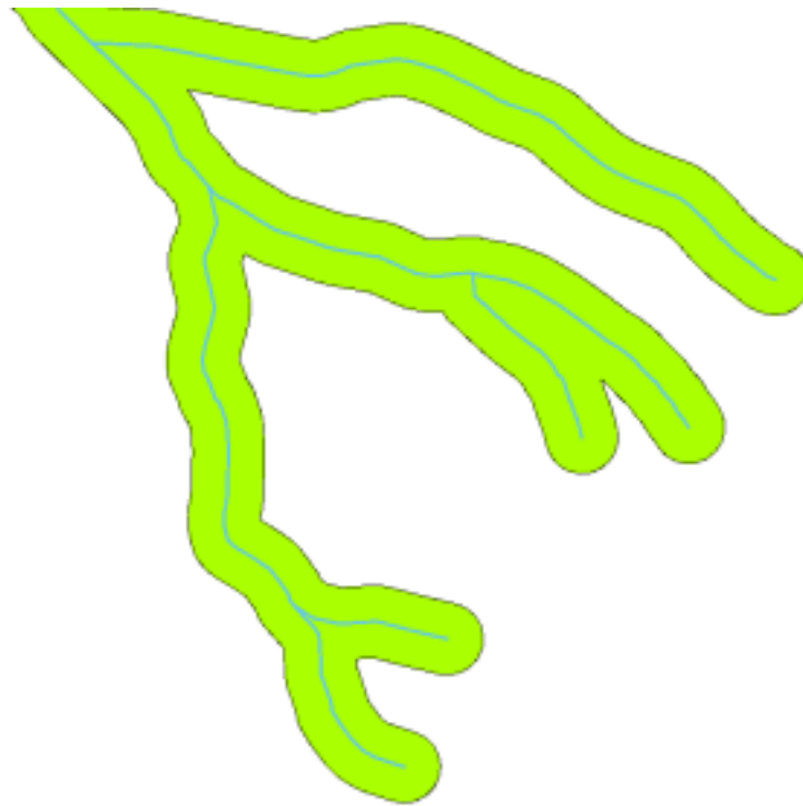
図 10.3: ベクタポリライン周辺のバッファゾーン。
