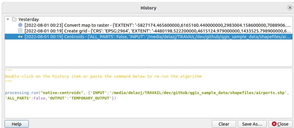
図 27.17: 履歴
