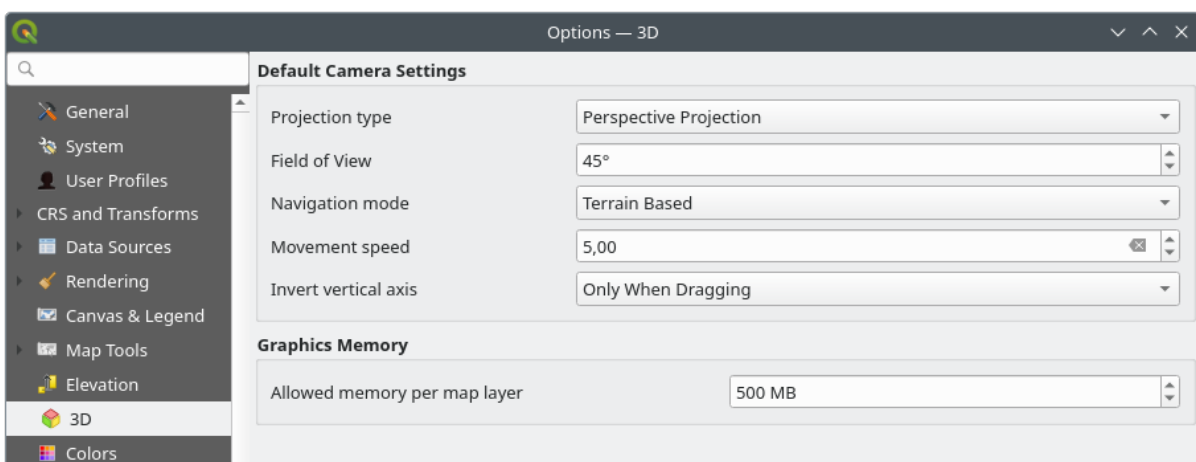
図 9.17: 3D の設定
