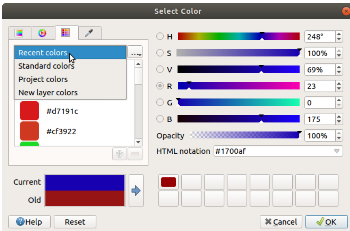
図 12.18: 色見本タブ
