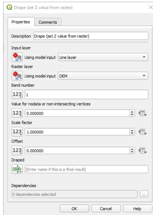
Fig. 27.23: Parametri in ingresso e in uscita dell'algorithmo
