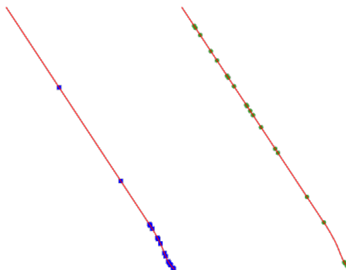
Figure28.51: Exemple de sortie d'algorithme. A gauche : points aléatoires le long de la ligne , à droite : points aléatoires sur les lignes ,
