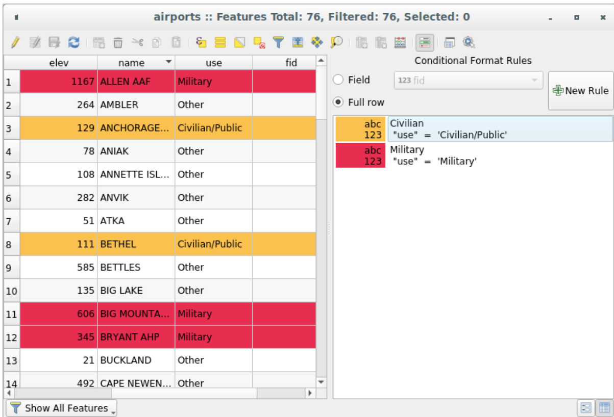
Abb. 16.69: Bedingte Formatierungsregeln für Attributtabelle
