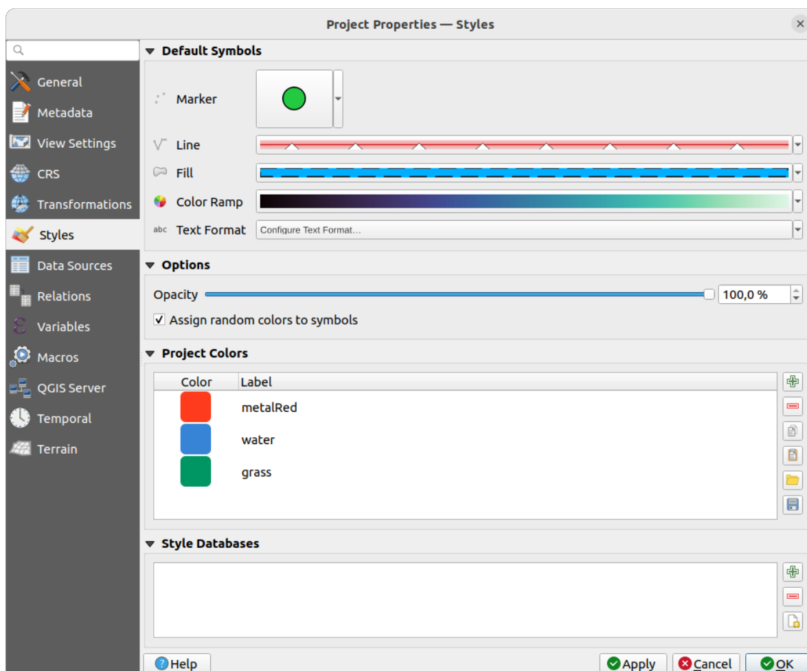
Abb. 9.34: Styles tab
