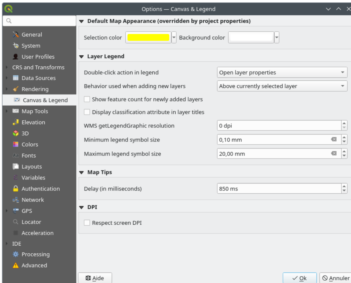
Abb. 9.13: Optionen auf dem Karte und Legende Reiter
