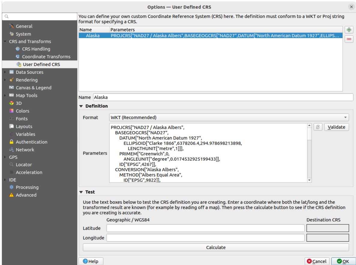
Abb. 9.5: Benutzerdefinierte KBS
