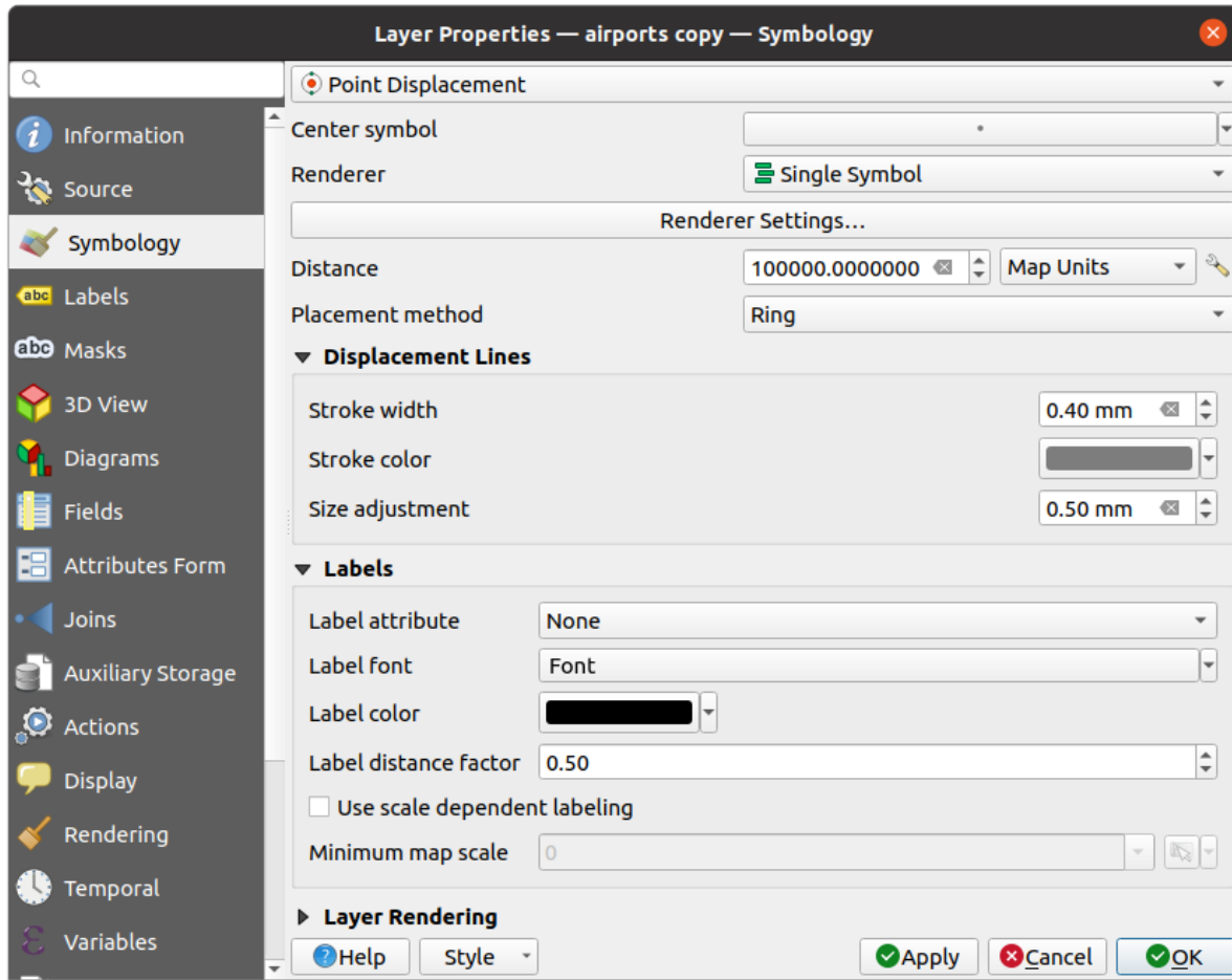
Abb. 16.8: Dialog Punktverdrängung
